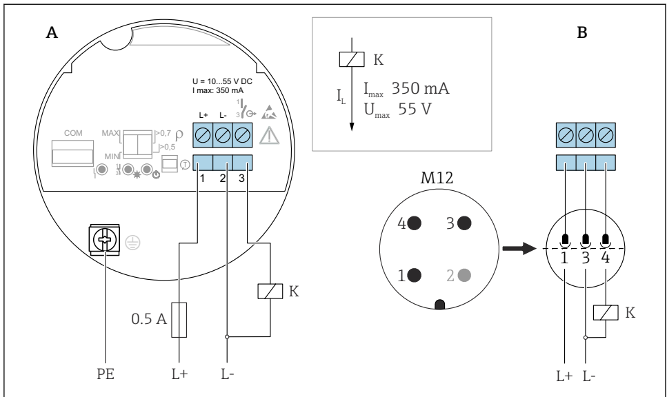
16 3 vezetékű DC-PPV, FEL62 elektronikus betét
