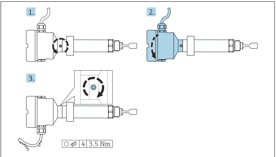
11 Ház külső rögzítőcsavarral és cseppelvezető hurokkal
