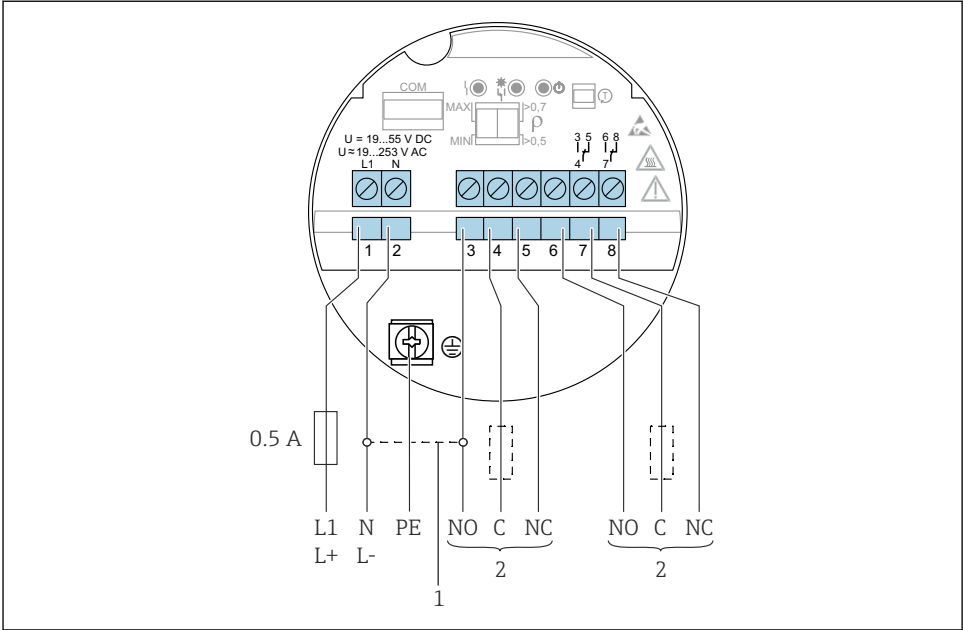
18 Connexion de courant universelle avec sortie relais, électronique FEL64
