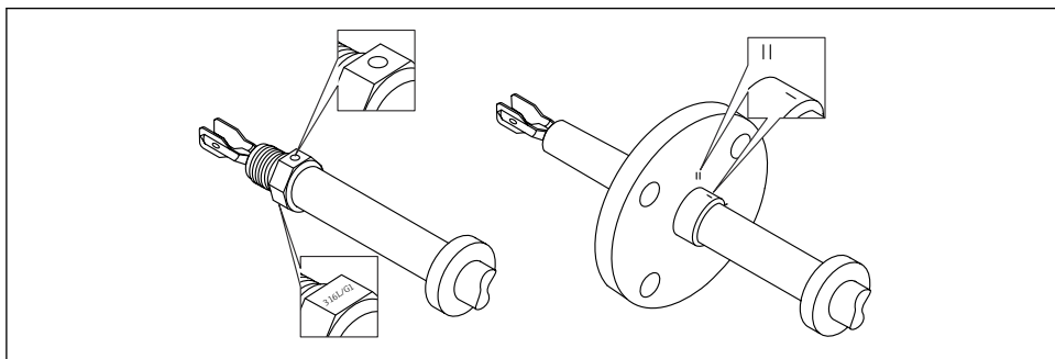
8 Poloha vibrační vidličky při vodorovné instalaci v nádobě pomocí označení
