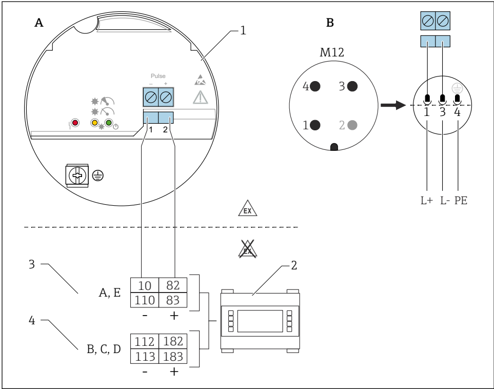
16 Diagrama de conexiones: conexión del módulo del sistema electrónico FEL60D al calculador de densidad FML621
