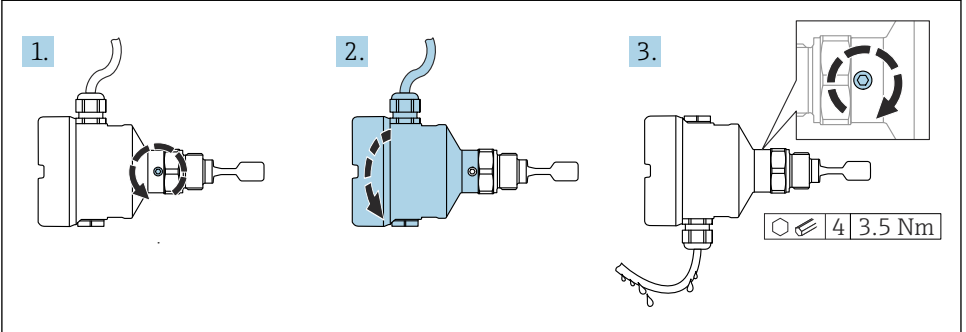
14 Harici kilit vidası ve damlama döngüsüne sahip muhafaza
