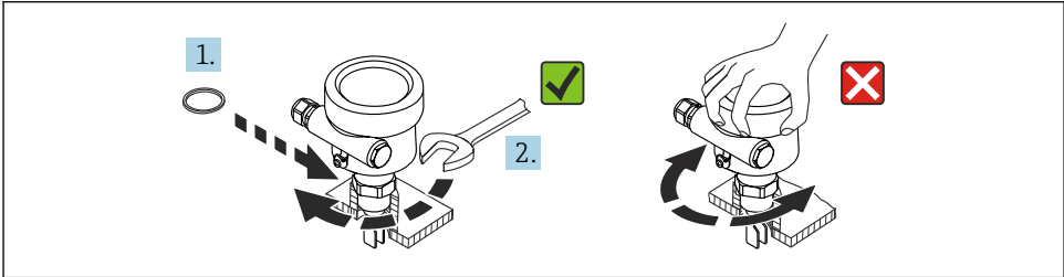
12 Cihazın vidalanması
