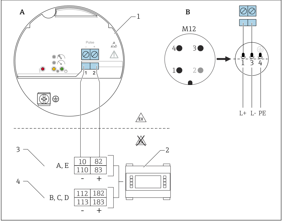
16 Bağlantı şeması: elektronik parça FEL60D'nin Yoğunluk Bilgisayarı FML621'e bağlantısı
