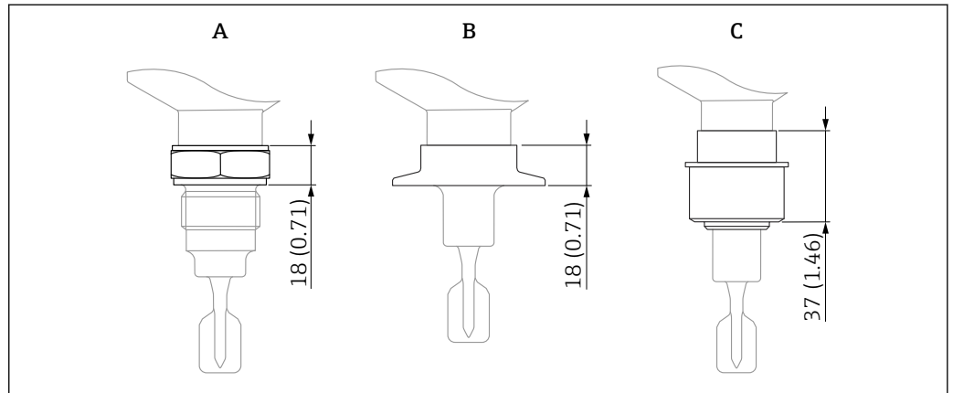
图 41 过程连接的最大高度规格。测量单位 mm (in)
