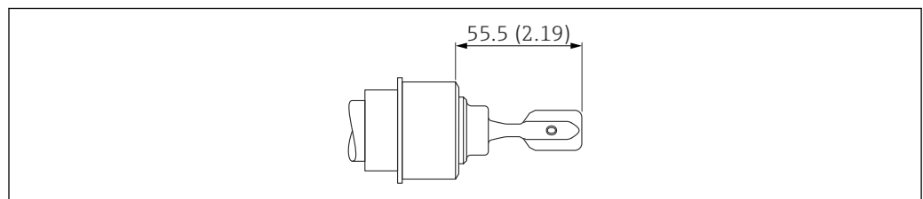
图 45 罐体接头（齐平安装在焊座中）。测量单位 mm (in)
