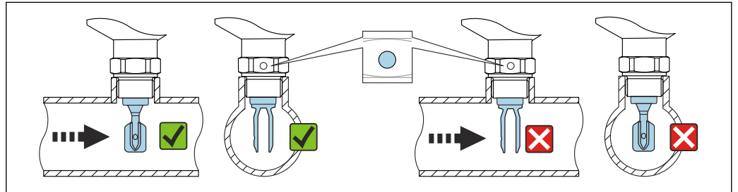
图 25 安装在管道中（注意叉体安装位置和标记）
