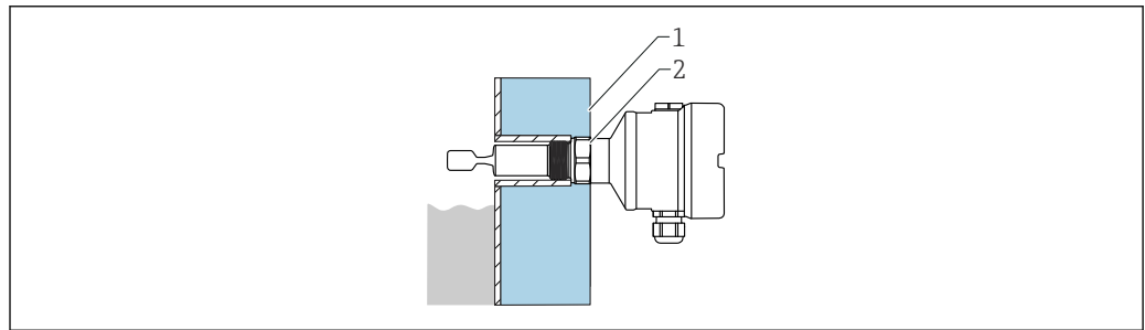
图 28 带保温层的罐体（实例）
