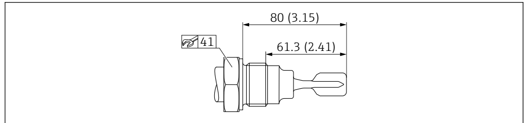
图 43 ISO228 G 1 螺纹。测量单位 mm (in)
