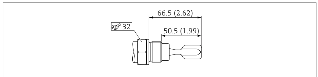
图 42 ISO228 G ¾螺纹。测量单位 mm (in)
