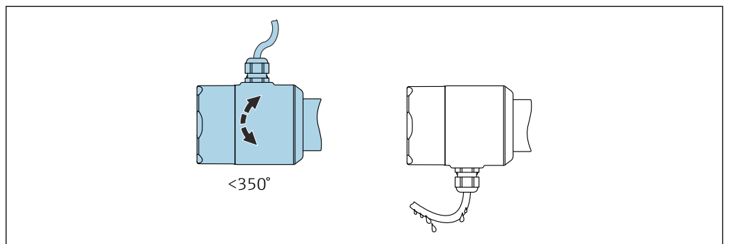
图 26 外壳不带锁紧螺丝，带排水回路
