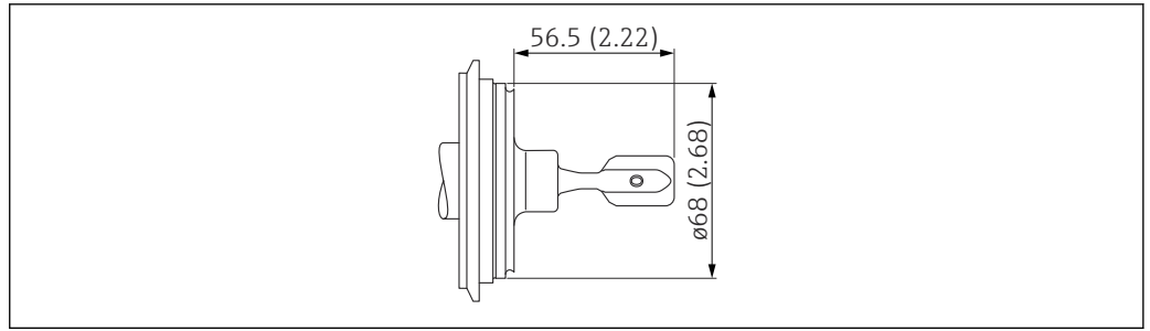
50 Varivent N 型接头, DN65-162 PN25 配合管道。测量单位 mm (in)
