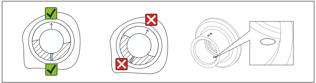
图 30 焊座，带泄漏检测孔
