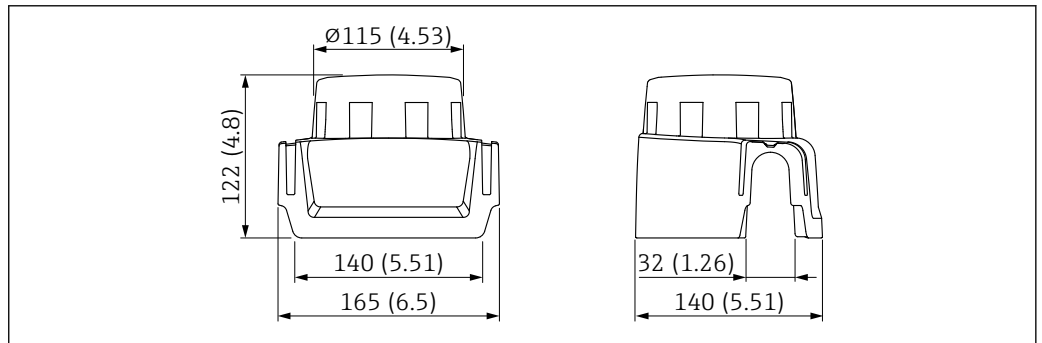
62 防护罩, 适用单腔体铝外壳。测量单位 mm (in)
