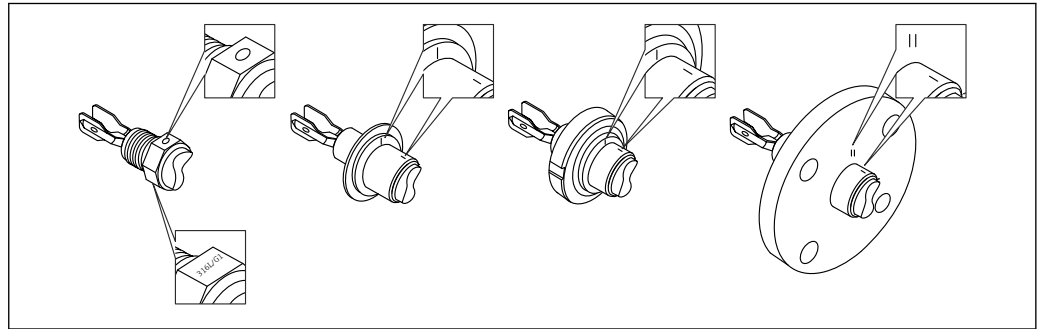
图 24 参照标记水平安装在罐体中的叉体位置
