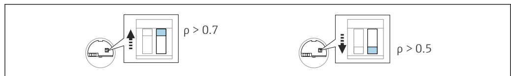
图 55 电子插件上的密度设置开关
