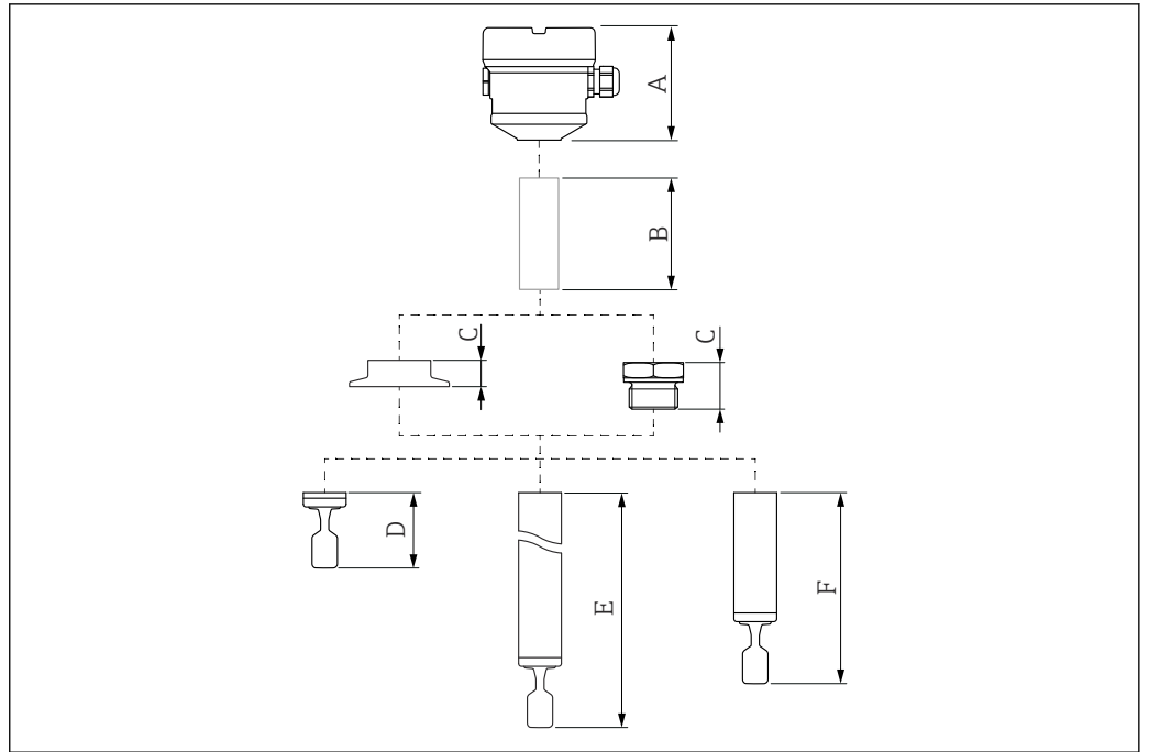
图 32 计算设备高度所需考虑的部件
