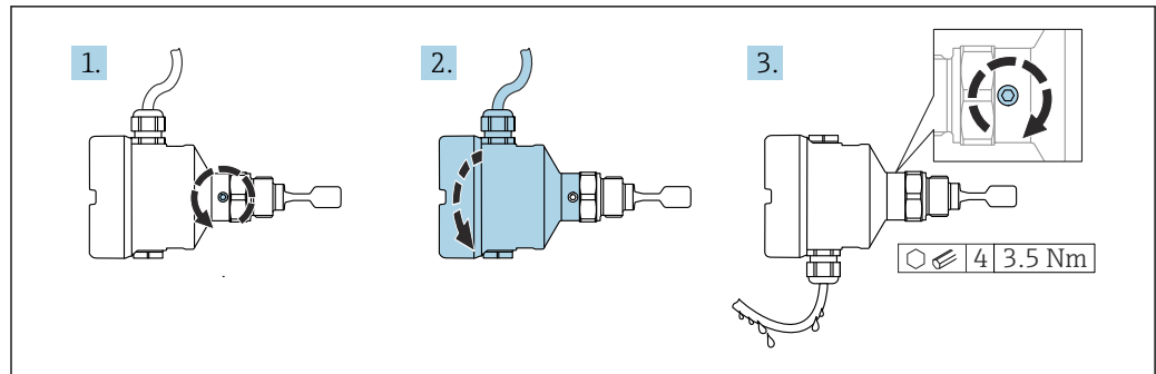
图 27 外壳带外部锁紧螺丝和排水回路
