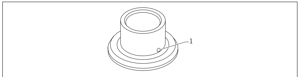
63 焊座, 带泄漏检测孔 (示意图)
