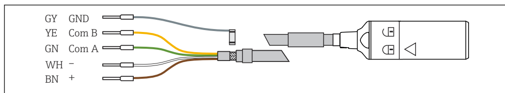
6 Измерительный кабель CYK10
