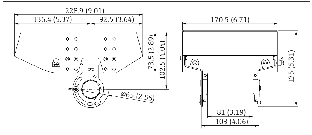
38 Dimensioni. Unità di misura mm (in)
