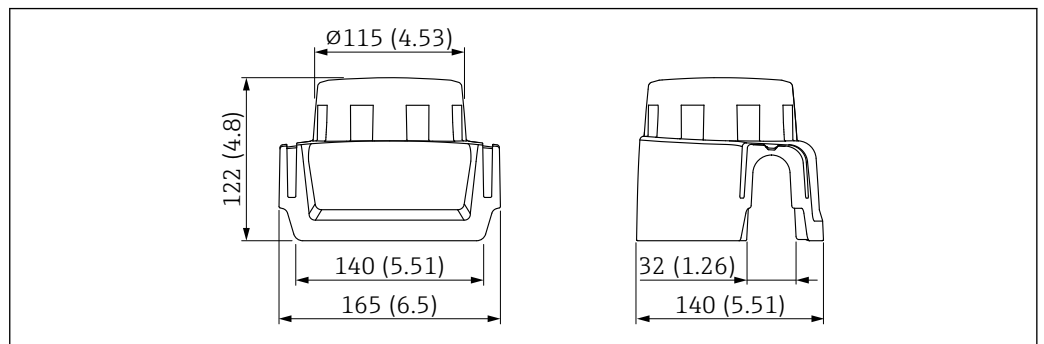
39 Dimensioni. Unità di misura mm (in)
