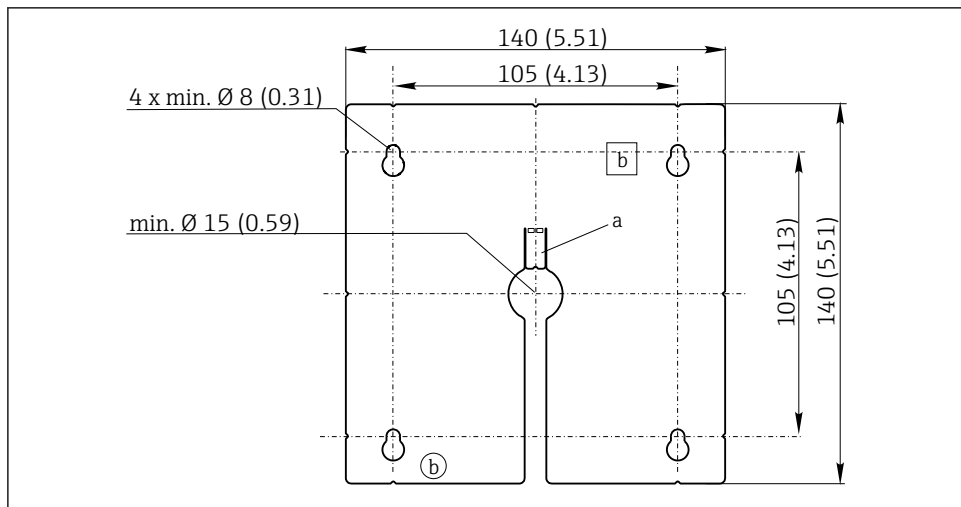
図 3 外部ディスプレイの取付プレート、寸法単位：mm (in)
