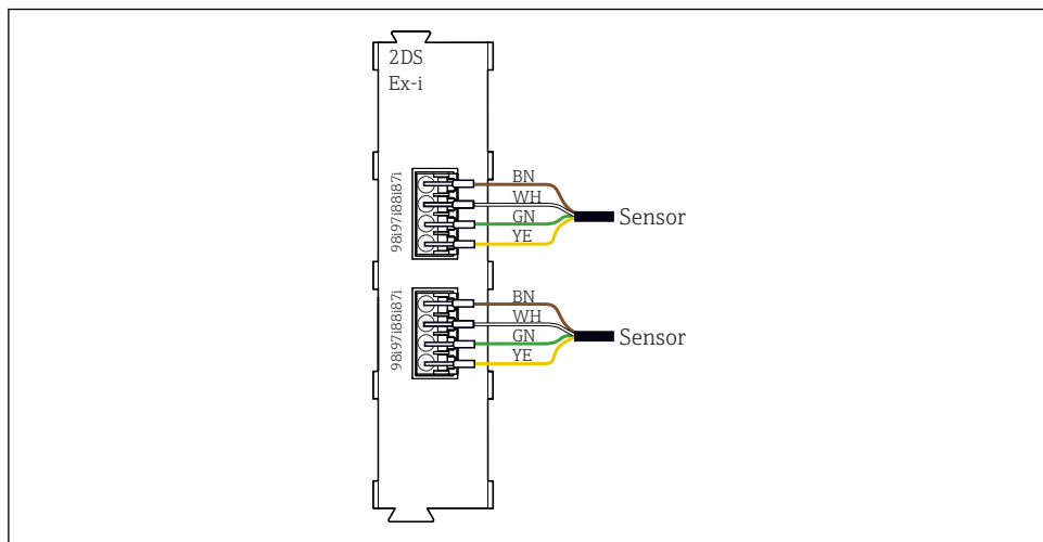
図 14 センサ通信モジュールタイプ 2DS Ex-i における追加の電源電圧のないセンサ
