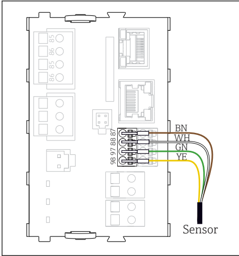
11 センサ、追加供給電圧なし
