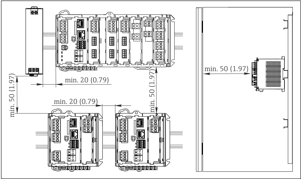
図 1 最小間隔 mm (in)
