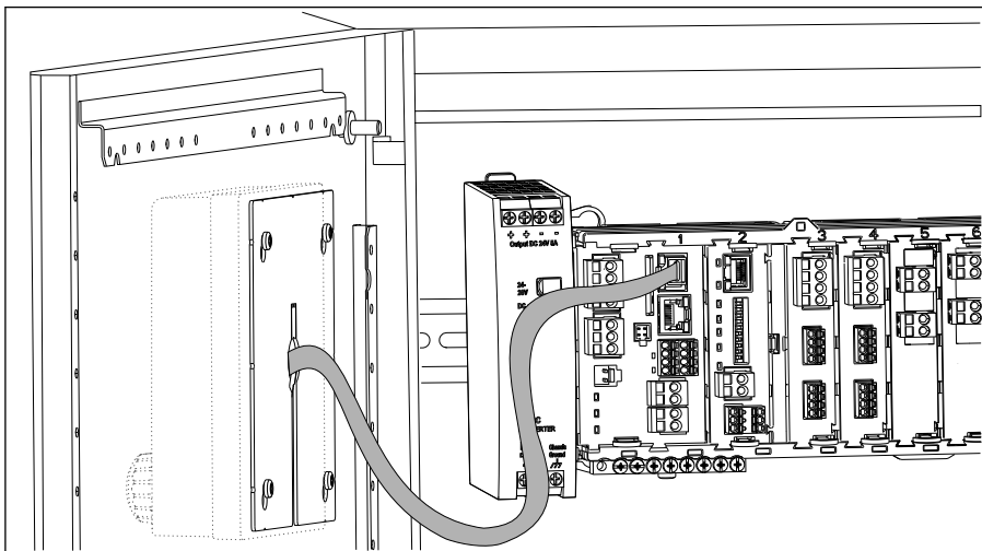
図 5 取付けが完了したディスプレイ
