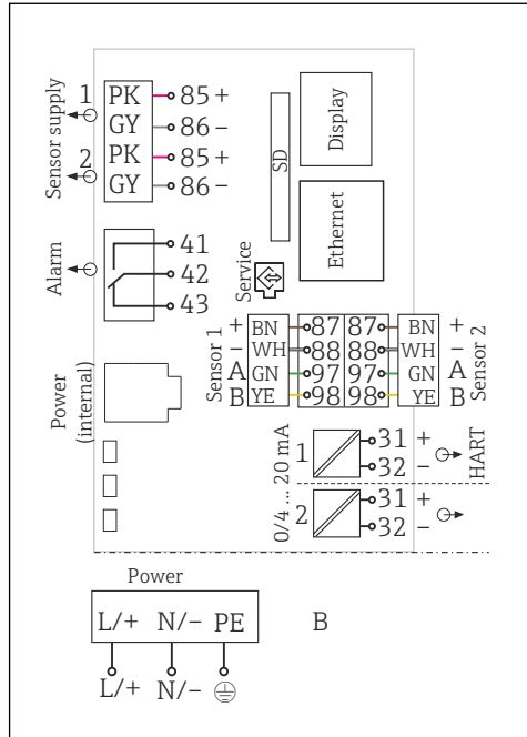
図 9 BASE2-E および外部電源ユニット (B) を使用した全体配線図例
