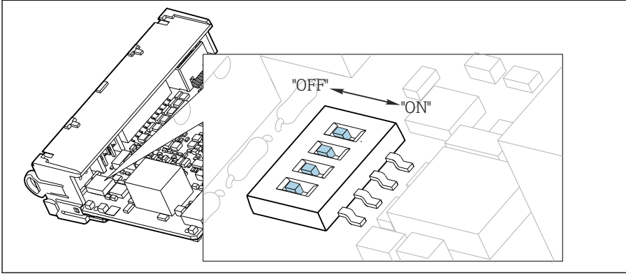
図 31 内部終端処理用の DIP スイッチ
