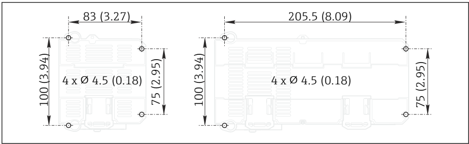
図 2 壁面取付の穴あけパターン mm (in)
