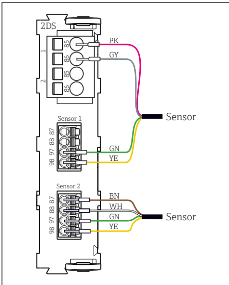
13 センサモジュール 2DS における追加供給電圧付きセンサと追加供給電圧なしのセンサ
