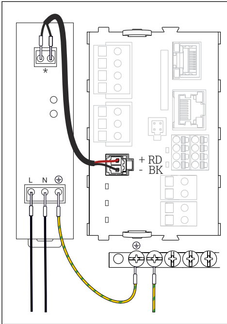
図 8 BASE2-E を使用した電源の接続例
