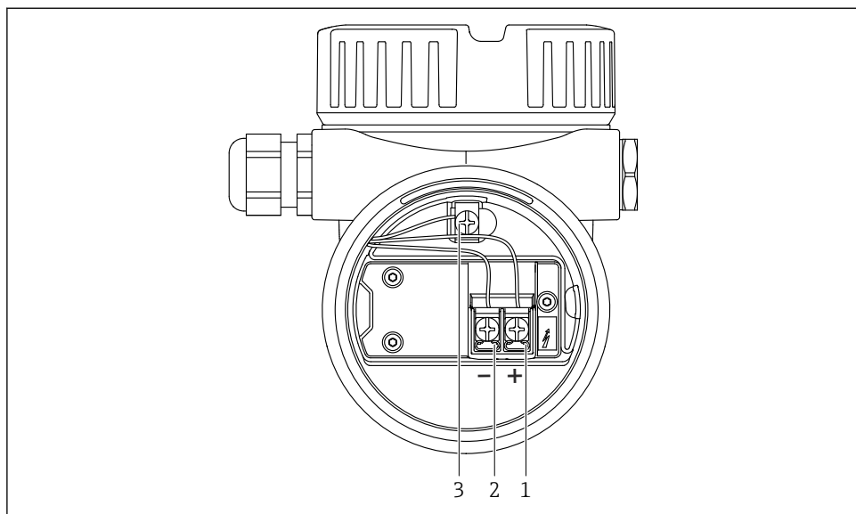
5 Terminales de conexión y borne de tierra en el compartimento de conexiones
