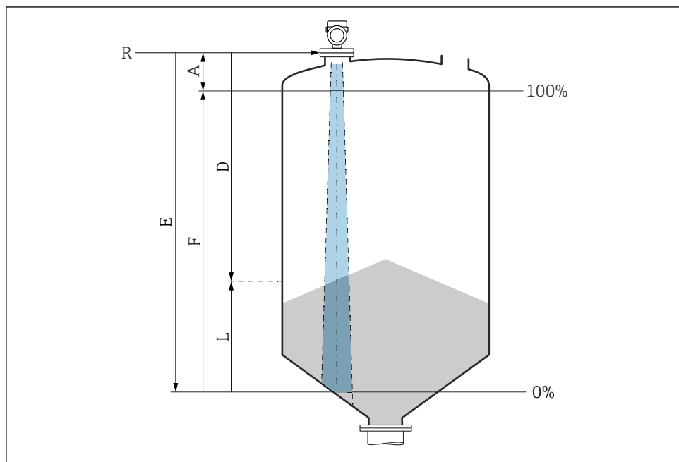
6 Parámetros de configuración para la medición de nivel en sólidos granulados
