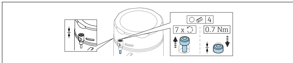
2 Cubierta con tornillo de fijación; caja higiénica (solo para protección contra explosiones por polvo)
