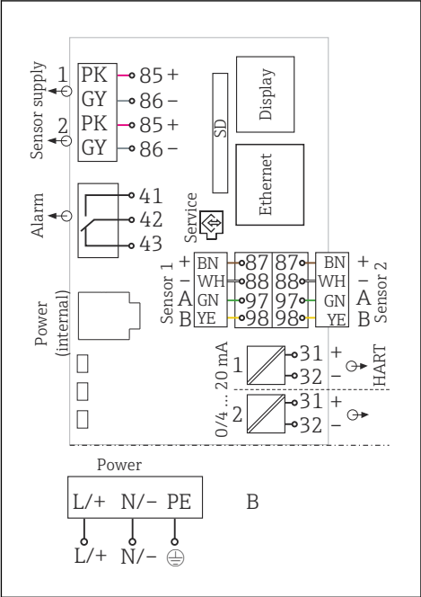
25 Diagrama de ligação elétrica completo usando o exemplo do BASE2-E e unidade de fonte de alimentação de extensão (B)
