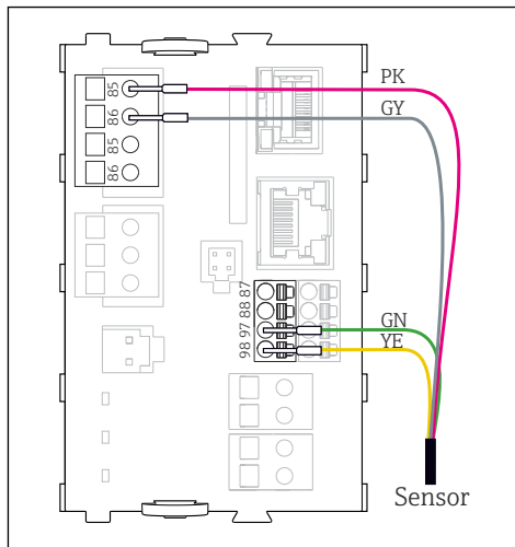
31 Sensores Memosens com fonte de alimentação adicional
