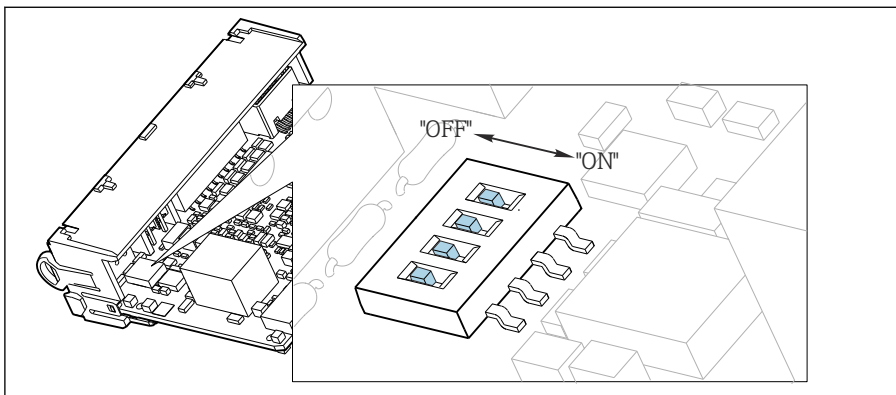
61 Minisseletora para terminação interna
