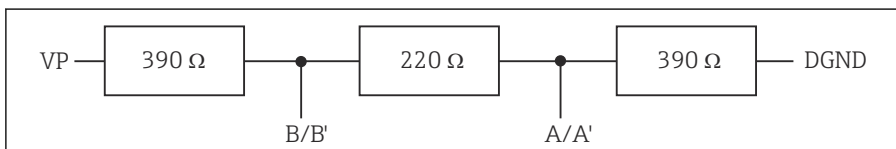
62 Estrutura da terminação interna
