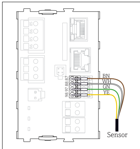
30 Sensores Memosens sem fonte de alimentação adicional
