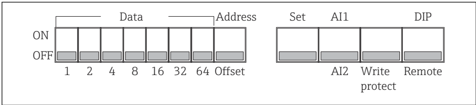
11 Nastavev stikal DIP
