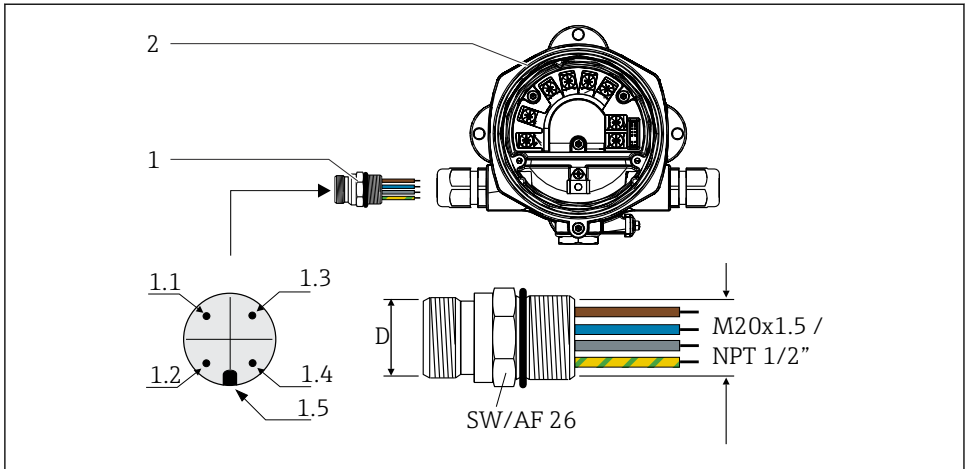
7 Konektorji za priključitev na procesno vodilo PROFIBUS® PA
