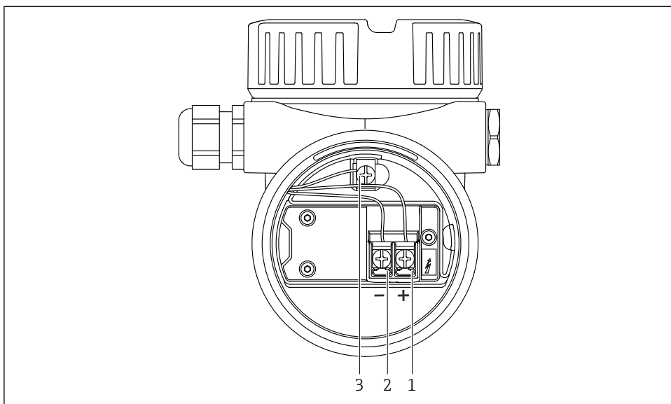
▣ 17 Bornele de conexiune și borna de împământare din compartimentul de conexiuni
