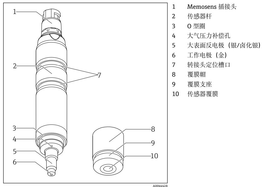
图 1 传感器结构
