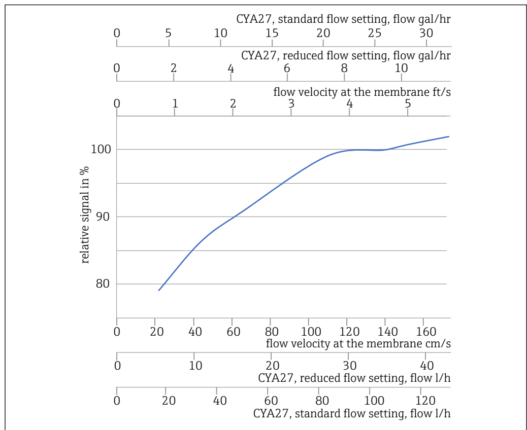
图 2 电极斜率与覆膜处流速/安装支架中流量的相互关系
