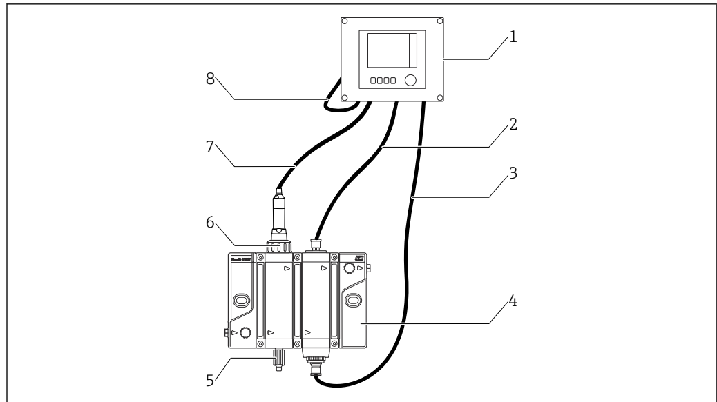
图 4 测量系统示意图
