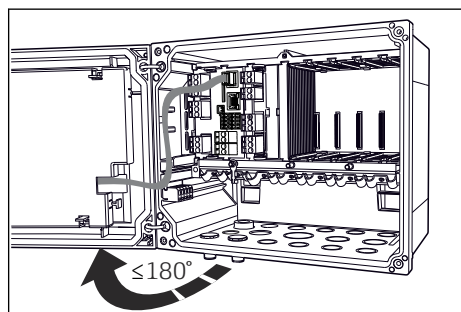
14 Ouvrir le couvercle de l'afficheur, angle d'ouverture max. 180° (dépend de la position de montage)
