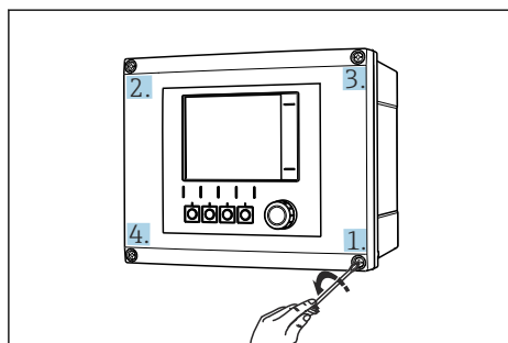
13 Desserrer les vis du boîtier en croix avec un tournevis cruciforme.
