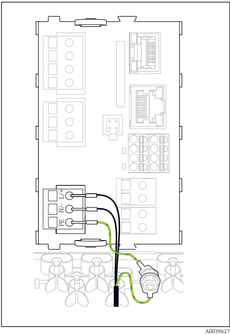
19 Raccordement de l'alimentation, exemple du BASE2-H ou -L
