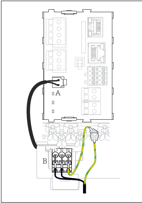
22 Raccordement de l'alimentation, exemple du BASE2-E
