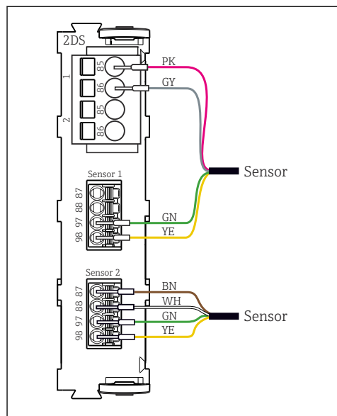
27 Capteurs avec et sans tension d'alimentation supplémentaire sur le module capteur 2DS
