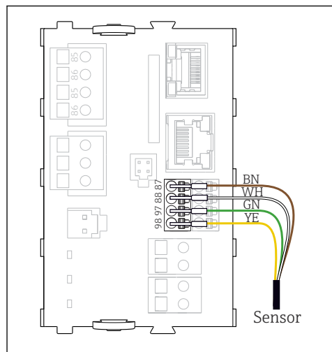
25 Capteurs sans tension d'alimentation supplémentaire
