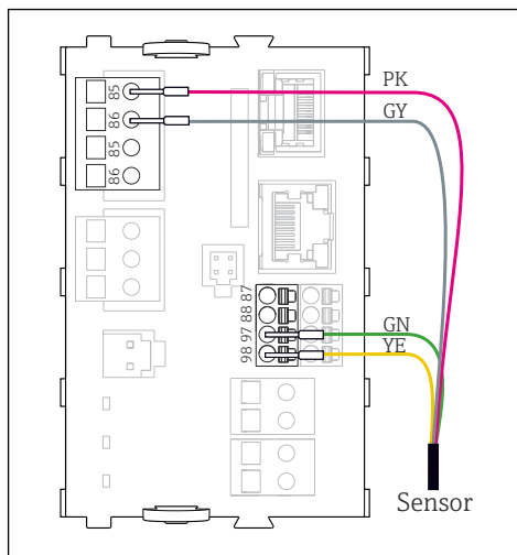
26 Capteurs avec tension d'alimentation supplémentaire
