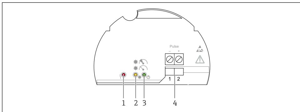
図 19 エレクトロニックインサート FEL60D
