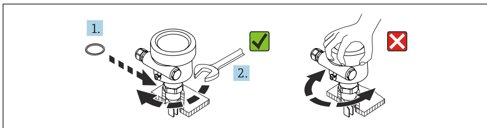
図 12 機器のネジ止め
