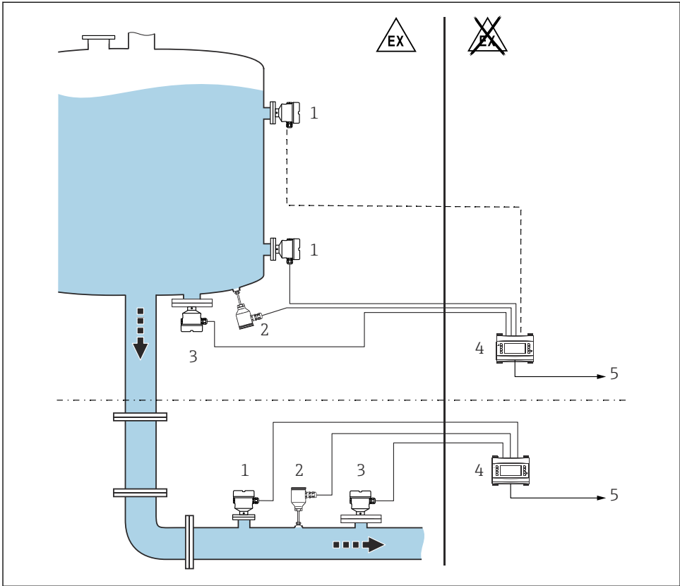
図 17 デンシティコンピュータ FML621 を使用した密度測定
