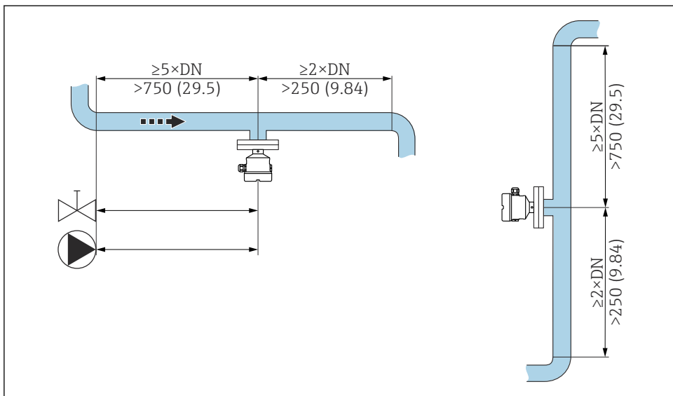
図 5 上流側直管長の取付け。測定単位 mm (in)
