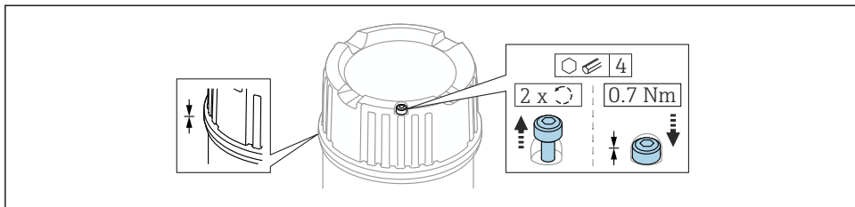
図 15 固定ねじ付きカバー
