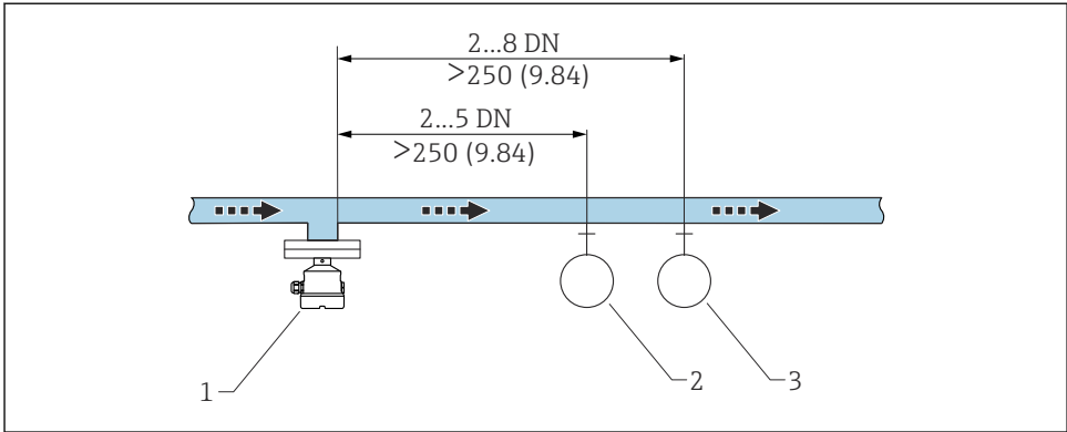
図 6 下流側直管長の取付け。測定単位 mm (in)
