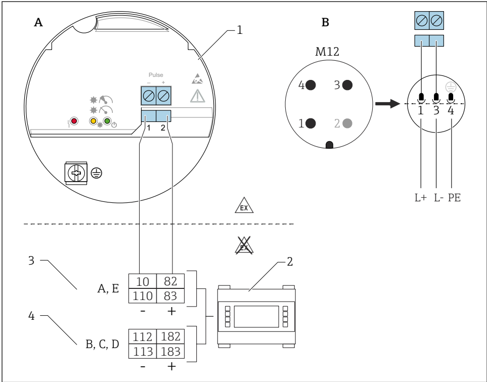
図 16 接続図：エレクトロニックインサート FEL60D とデンシティコンピュータ FML621 の接続
