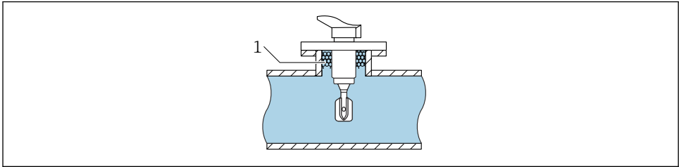
図 3 パイプ内の測定物の流れの中への設置例
