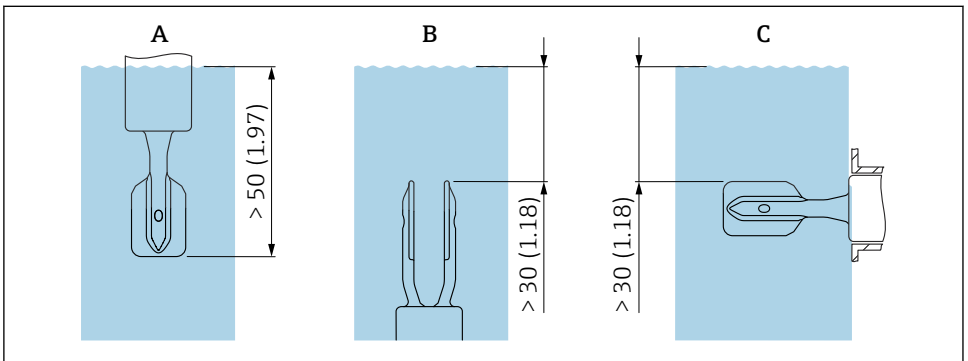
図 2 単位 mm (in)
