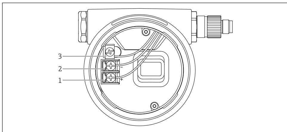
图 3 接线腔中的接线端子和接地端
