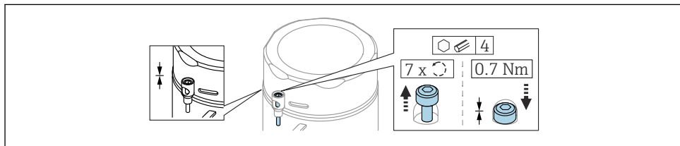
图 2 带锁定螺丝的外壳盖；卫生型外壳（仅适用粉尘防爆场合）
