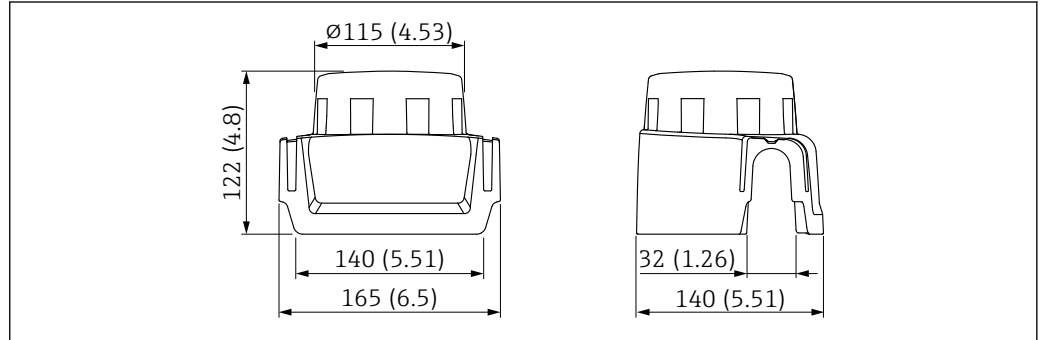
图 68 外形尺寸示意图。测量单位 mm (in)
