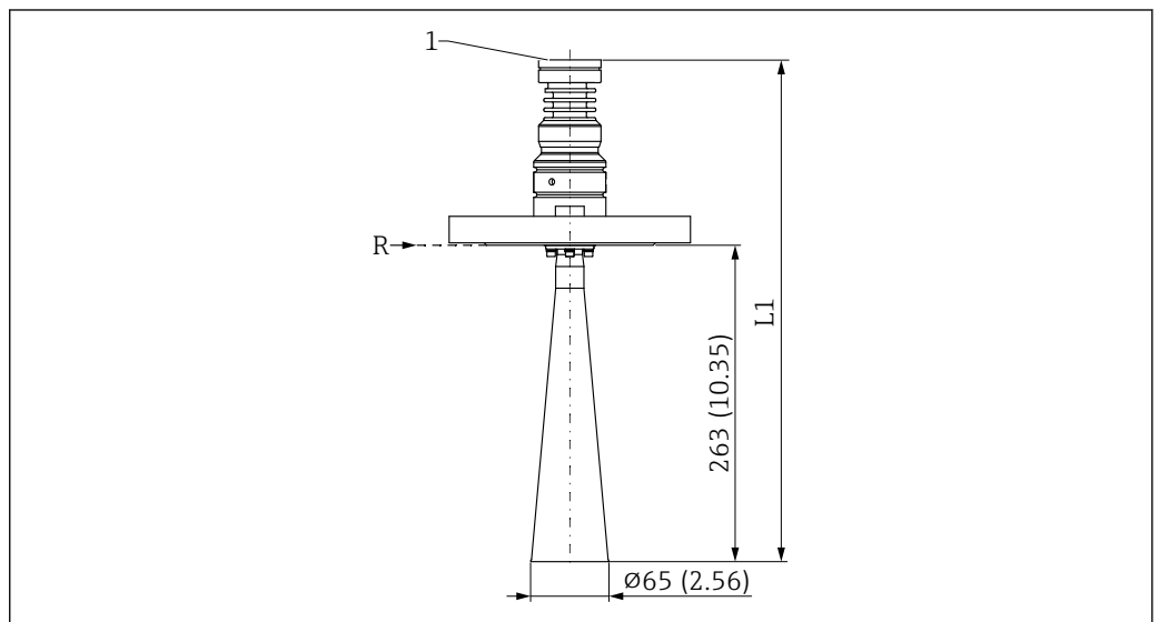
图 57 DN65 喇叭天线的外形尺寸示意图; 法兰过程连接。测量单位 mm (in)
