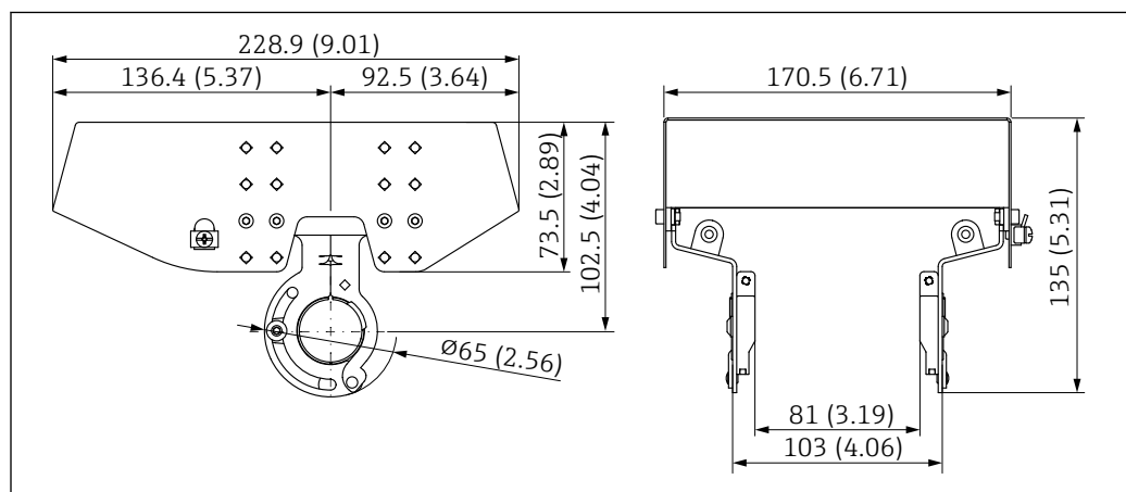
图 67 外形尺寸示意图。测量单位 mm (in)
