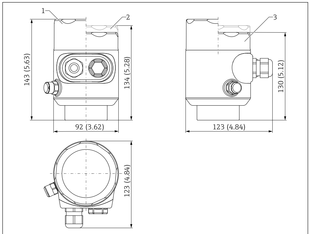
图 54 316L 单腔室外壳 (卫生型) 的外形尺寸示意图。测量单位 mm (in)
