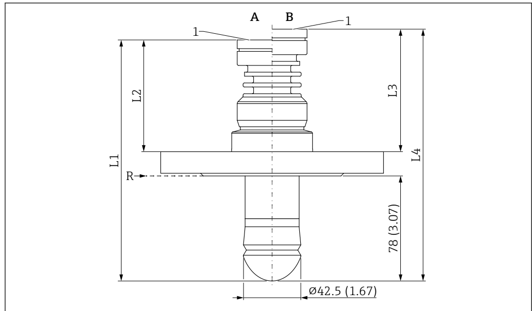
图 58 法兰过程连接的外形尺寸示意图。测量单位 mm (in)
