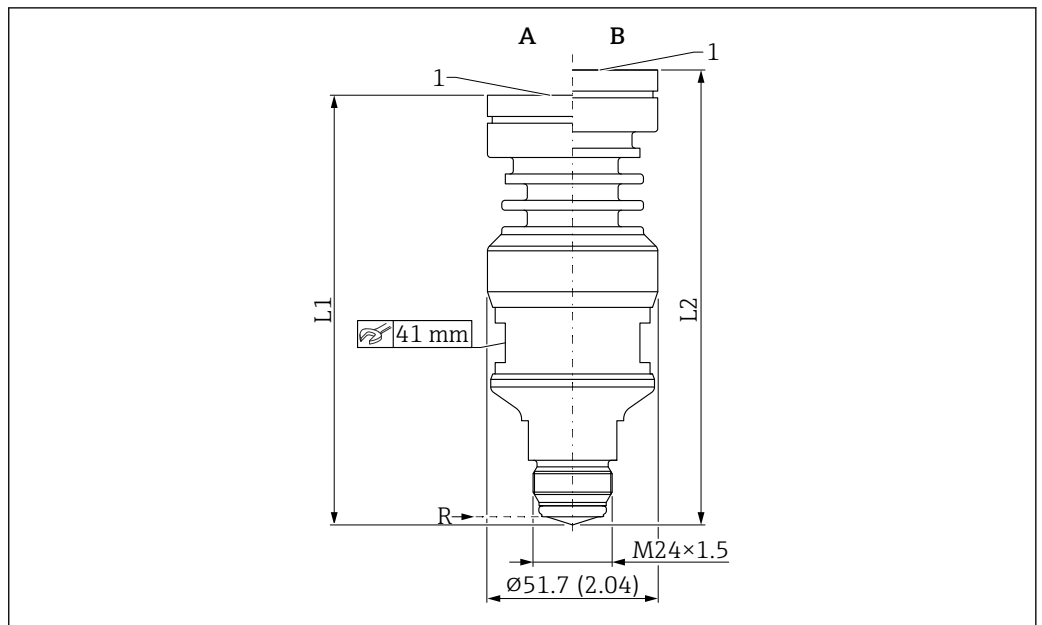
35 PEEK 一体式天线（20 mm 口径）的外形尺寸示意图；M24×1.5 过程连接。测量单位 mm (in)
