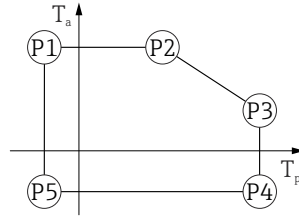
图 22 316L 外壳; 过程温度范围: -20 ... +150 °C (-4 ... +302 °F)
