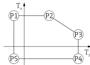
图 29 316L 外壳，卫生型；过程温度范围：-40 ... +200 °C (-40 ... +392 °F)
