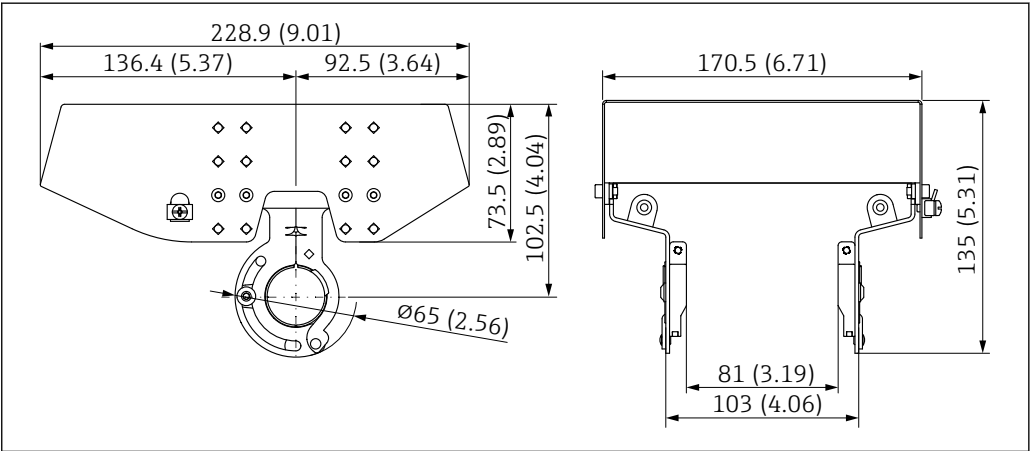
图 48 外形尺寸示意图。测量单位 mm (in)
