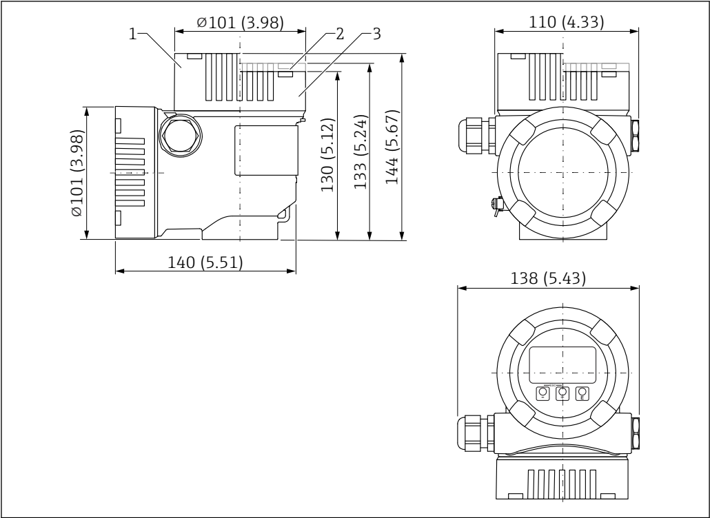
图 34 双腔室外壳 (L 型) 的外形尺寸示意图。测量单位 mm (in)
