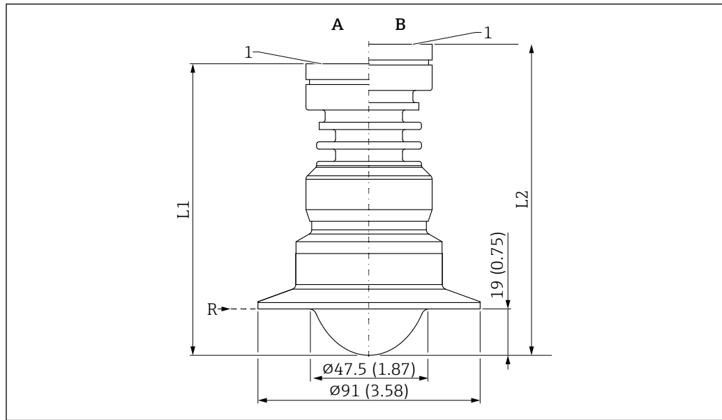
图 39 PTFE 涂层天线（齐平安装，50 mm (2 in)口径）的外形尺寸示意图；带 ISO2852 Tri-Clamp DN70-76.1 (3")卡箍。测量单位 mm (in)
