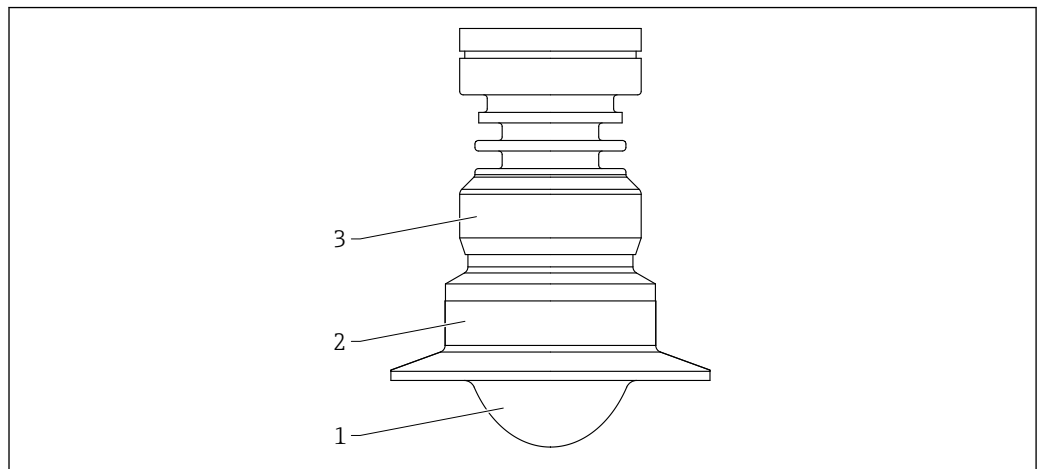
图 44 PTFE 涂层天线（齐平安装，50 mm (2 in)口径）的材质；带 ISO2852 Tri-Clamp 卡箍。测量单位 mm (in)
