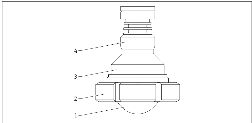
图 43 涂层天线（齐平安装，80 mm (3 in)口径）的材质；带 DIN11851 开槽螺母。测量单位 mm (in)
