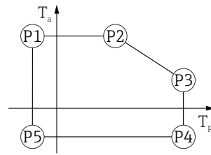
图 28 316L 外壳，卫生型；过程温度范围：-40 ... +150 °C (-40 ... +302 °F)
