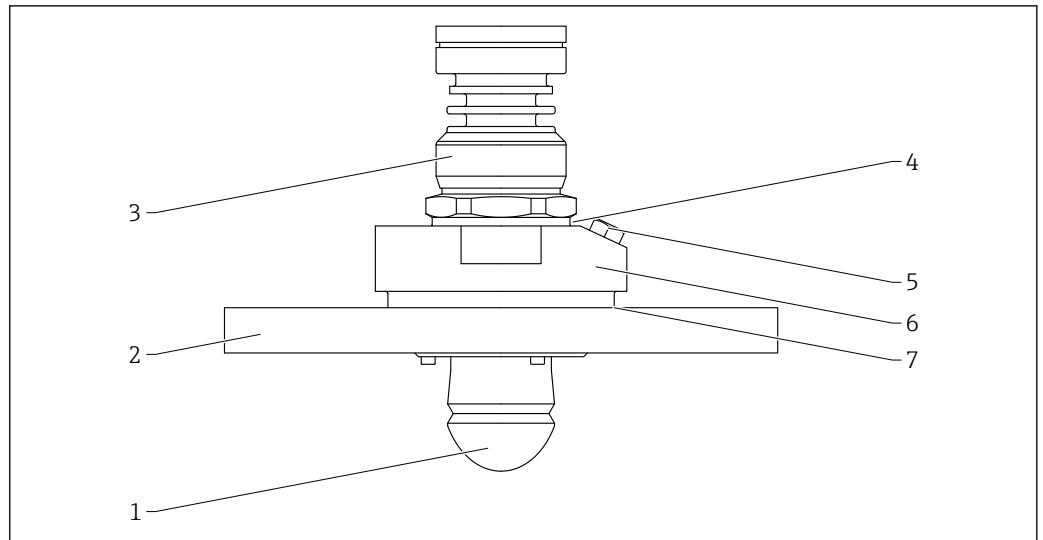
61 水滴型天线的材质；带空气吹扫接口。测量单位 mm (in)
