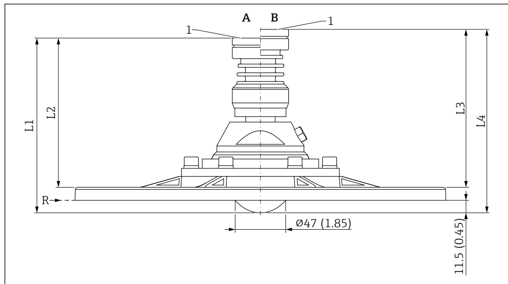
图 54 齐平安装天线 (80 mm (3 in) 口径) 的外形尺寸示意图; 带 UNI 法兰、天线角度调节装置和空气吹扫接口。测量单位 mm (in)
