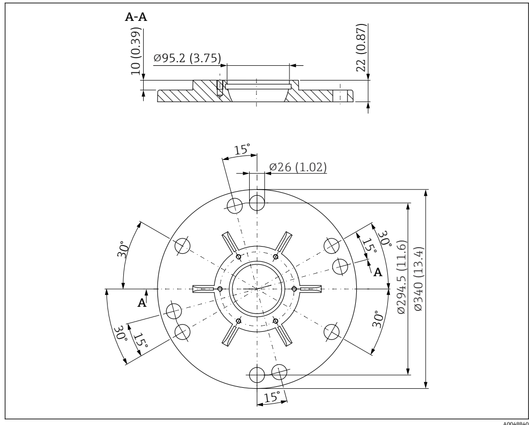
图 44 UNI 8"/DN200/200A 法兰的外形尺寸示意图；适用带天线角度调节装置的天线。测量单位 mm (in)
