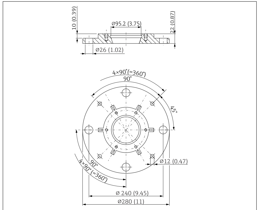
图 43 UNI 6"/DN150/150A 法兰的外形尺寸示意图；适用带角度调节装置的天线。测量单位 mm (in)
