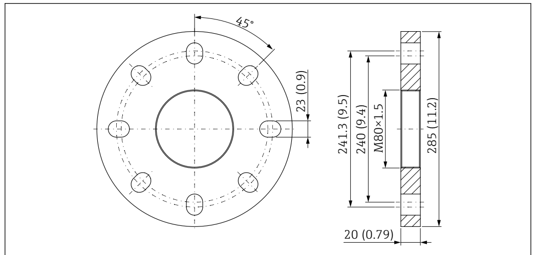
49 UNI 6"/DN150/150A 法兰, 适用带空气吹扫接口的 PTFE 水滴型天线 (50 mm (2 in) 口径)。测量单位 mm (in)
