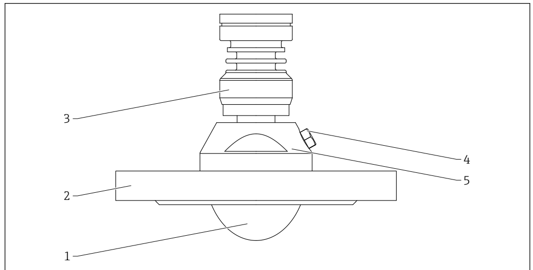
62 齐平安装天线（80 mm (3 in)口径）的材质；带法兰和空气吹扫接口。测量单位 mm (in)
