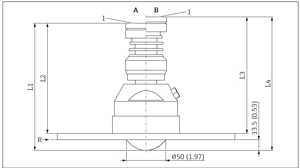
51 PTFE 齐平安装天线 (80 mm (3 in) 口径) 的外形尺寸示意图; 带 UNI 法兰和空气吹扫接口。测量单位 mm (in)
