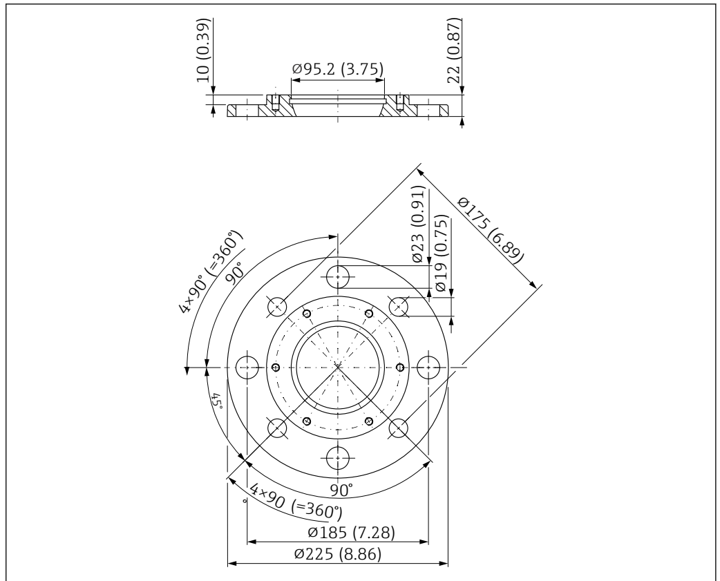
图 55 UNI 4"/DN100/100A 法兰的外形尺寸示意图; 适用带天线角度调节装置的天线。测量单位 mm (in)
