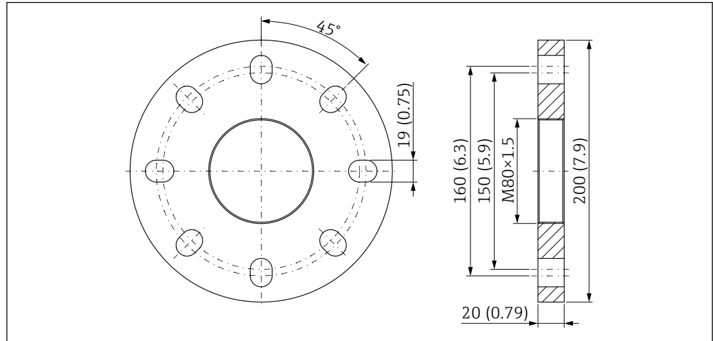
图 47 UNI 3"/DN80/80A 法兰, 适用带空气吹扫接口的 PTFE 水滴型天线 (50 mm (2 in)口径)。测量单位 mm (in)
