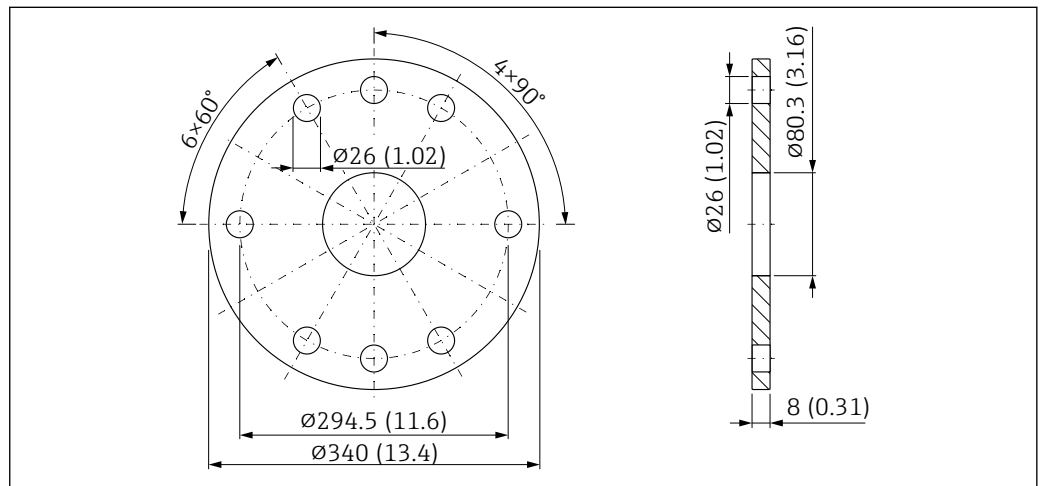
52 UNI 8"/DN200/200A 法兰的外形尺寸示意图; 适用带空气吹扫接口的 DN80 天线。测量单位 mm (in)
