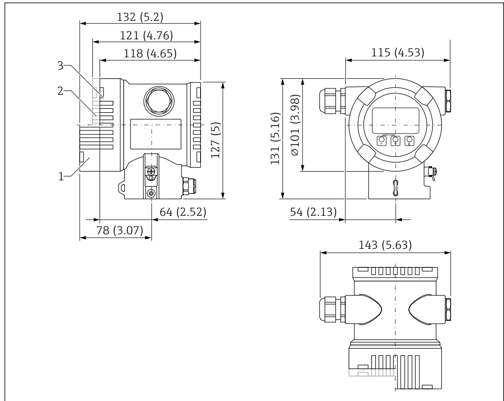
图 38 双腔室外壳的外形尺寸示意图。测量单位 mm (in)
