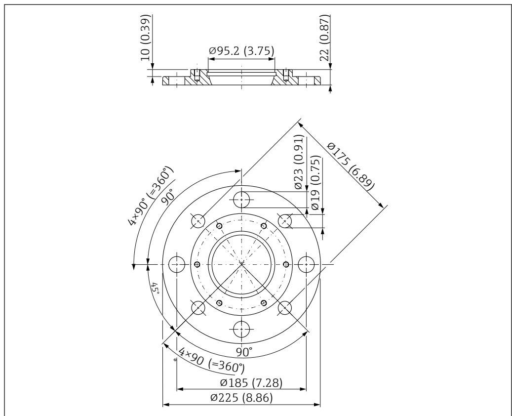
图 42 UNI 4"/DN100/100A 法兰的外形尺寸示意图；适用带天线角度调节装置的天线。测量单位 mm (in)
