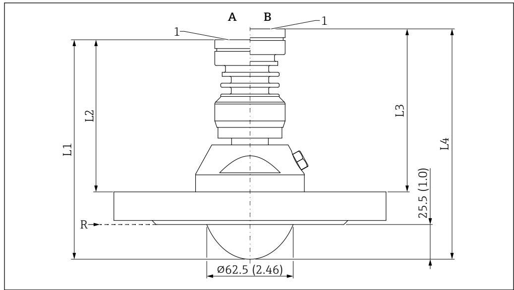
图 50 PTFE 齐平安装天线 (80 mm (3 in) 口径) 的外形尺寸示意图; 带标准法兰和空气吹扫接口。测量单位 mm (in)
