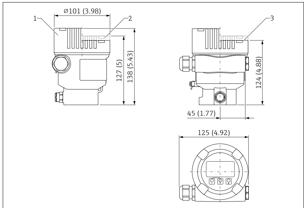
图 36 单腔室铝外壳的外形尺寸示意图。测量单位 mm (in)
