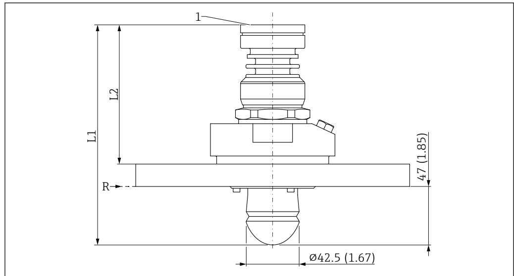
图 46 PTFE 水滴型天线 (50 mm (2 in)口径) 的外形尺寸示意图; 带 UNI 法兰和空气吹扫接口。测量单位 mm (in)
