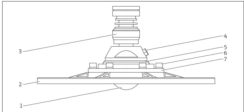
图 64 齐平安装天线 (80 mm (3 in)口径) 的材质; 带 UNI 法兰、天线角度调节装置和空气吹扫接口
