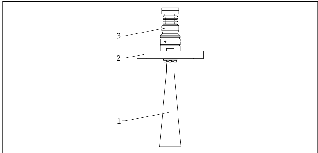
图 59 DN65 喇叭天线的材质。测量单位 mm (in)
