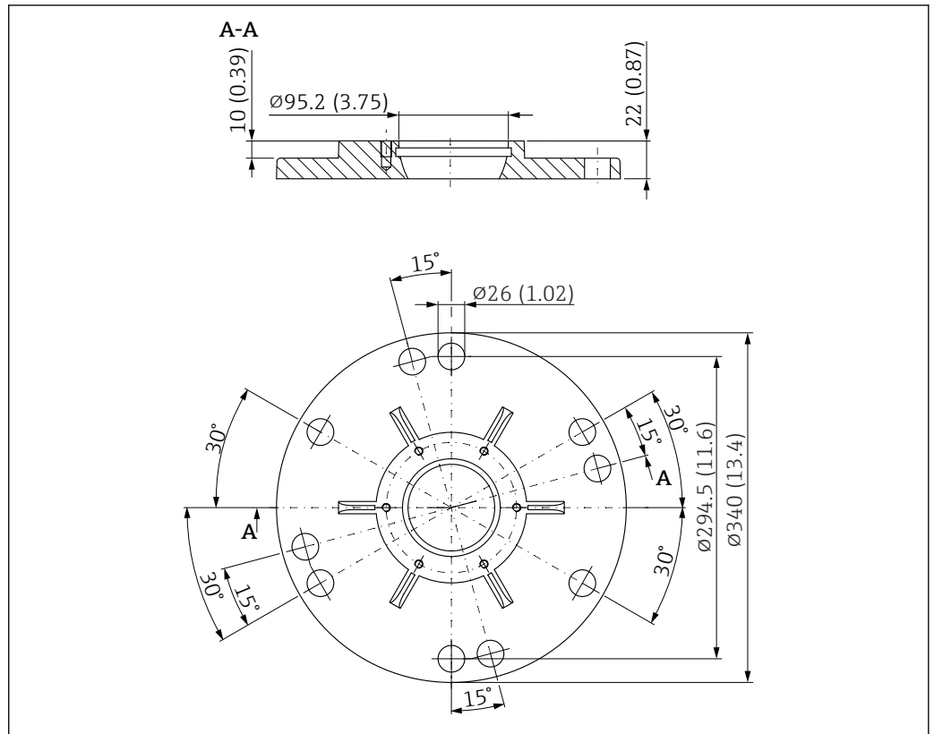
图 57 UNI 8"/DN200/200A 法兰的外形尺寸示意图；适用带天线角度调节装置的天线。测量单位 mm (in)
