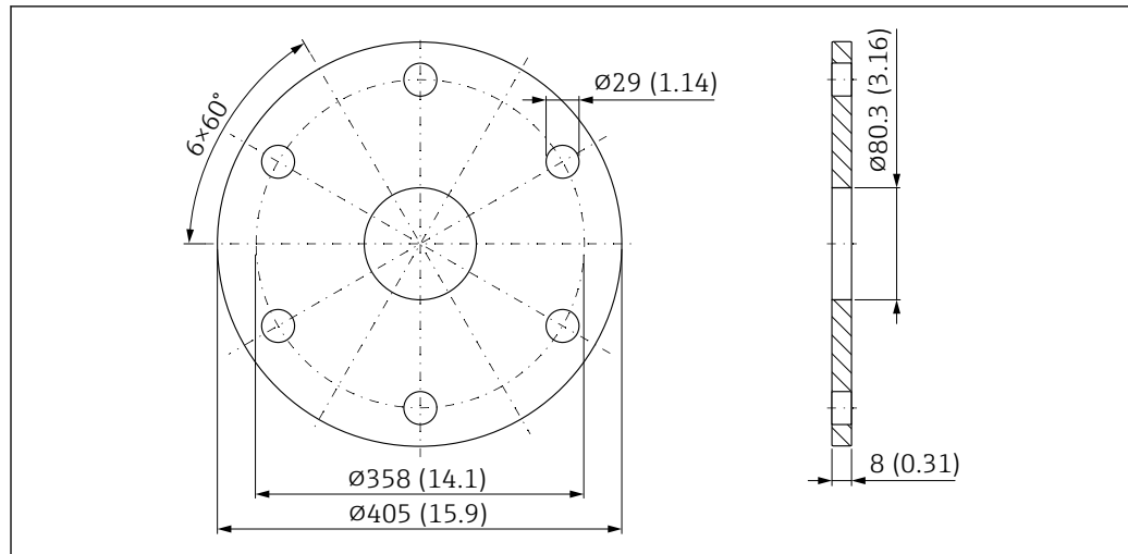
图 53 UNI 10"/DN250/250A 法兰的外形尺寸示意图; 适用带空气吹扫接口的 DN80 天线。测量单位 mm (in)
