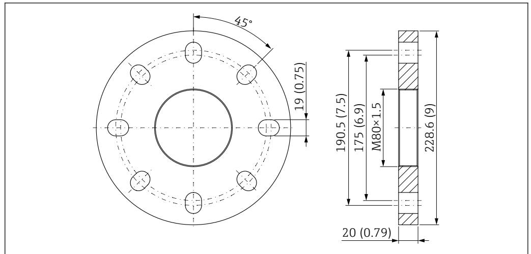
48 UNI 4"/DN100/100A 法兰, 适用带空气吹扫接口的 PTFE 水滴型天线 (50 mm (2 in) 口径)。测量单位 mm (in)
