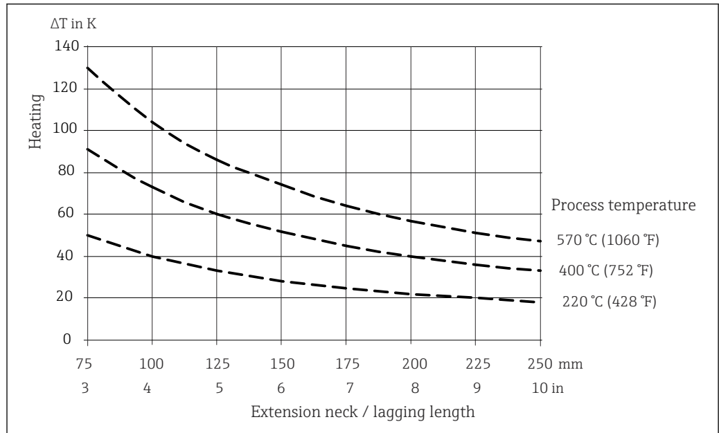
图 26 接线盒温度与过程温度的关系曲线。接线盒温度 = 环境温度 20 °C (68 °F) + ΔT
