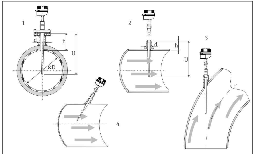
图 15 安装实例
