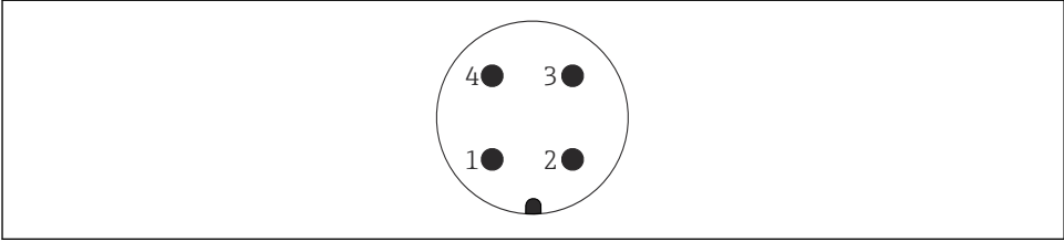
図 18 M12 プラグ、ピンの割当て
