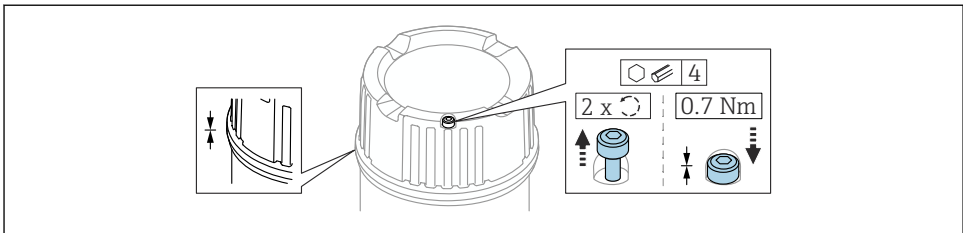
14 固定ねじ付きカバー
