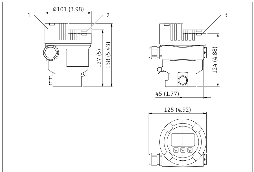
図 19 シングルコンパートメントハウジング、アルミニウムの寸法。測定単位 mm (in)
