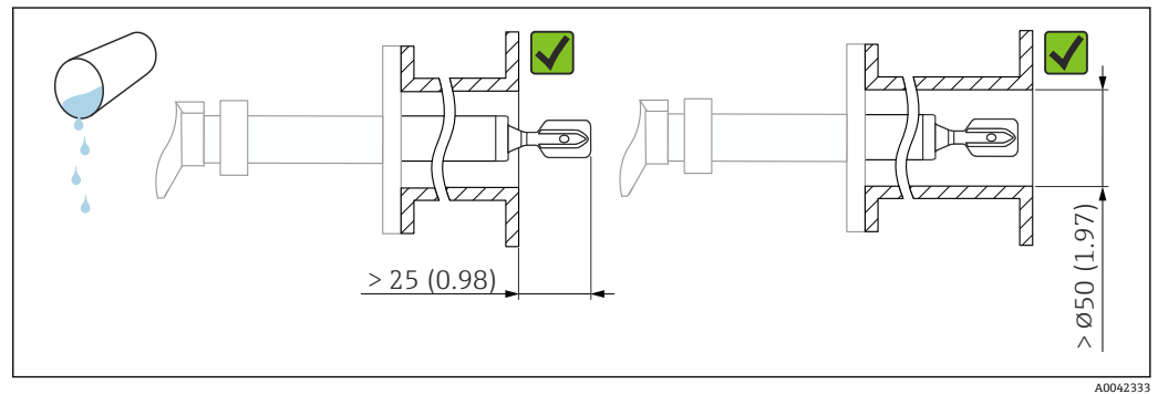
図 8 低粘度液体の設置例。測定単位 mm (in)
