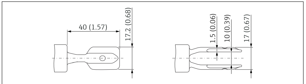
図 24 音叉部。測定単位 mm (in)
