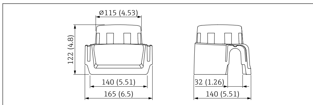
図 36 シングルコンパートメントハウジング用の保護カバー、アルミニウムまたは SUS 316L 相当。測定単位 mm (in)
