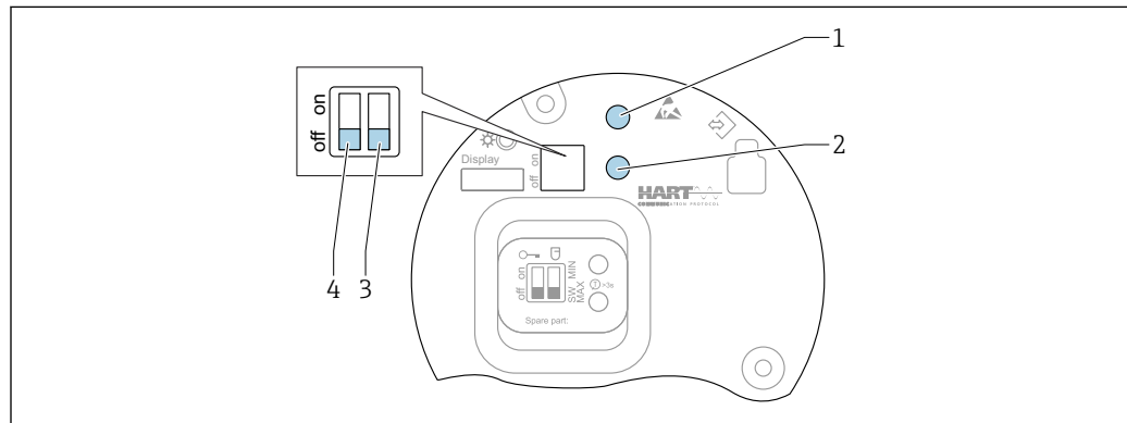
図 33 FEL60H エレクトロニックインサートの操作キーおよび DIP スイッチ
