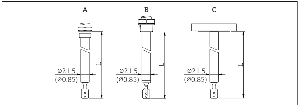
図 23 伸長パイプ (センサ長 L)。測定単位 mm (in)
