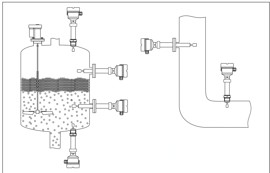
図 7 容器、タンク、またはパイプへの設置例
