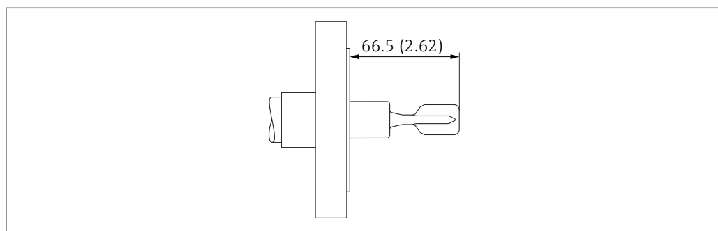
☑ 32 フランジ付きの例。測定単位 mm (in)
