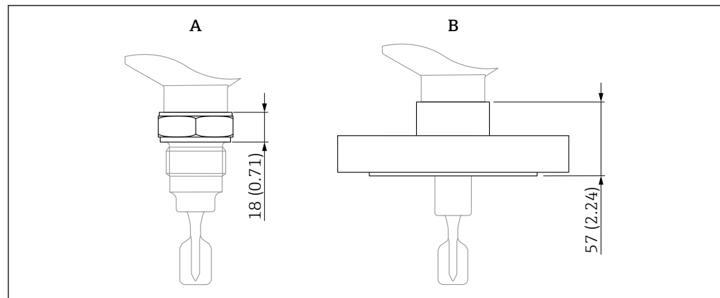
図 25 プロセス接続の最大高さ仕様
