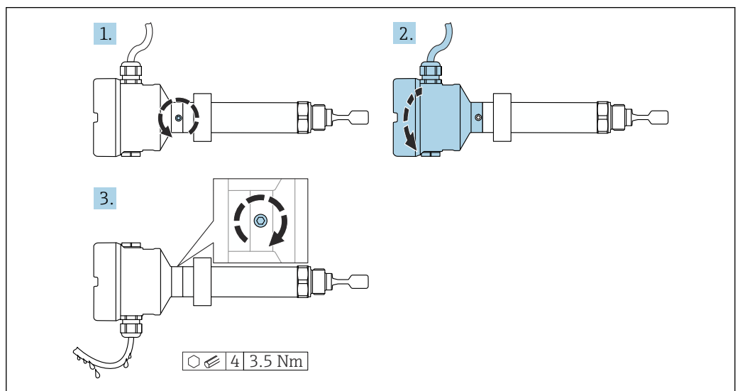
図 14 外部のロックネジおよびドリブループ付きハウジング
