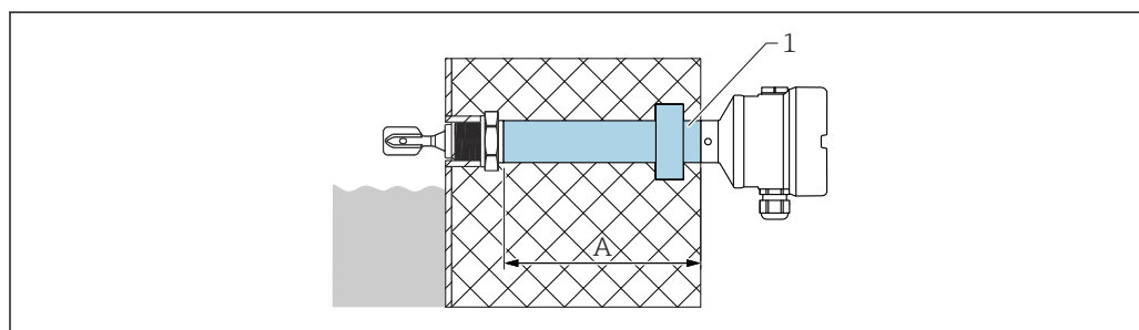
図 21 ガラスガスタイトフィードスルー付き温度セパレータ
