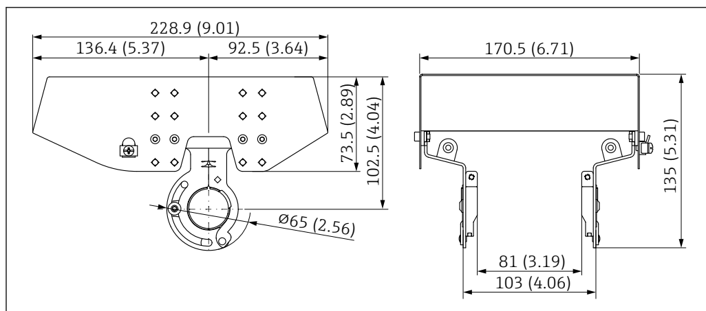
図 35 アルミニウム製デュアルコンパートメントハウジング用保護カバー。測定単位 mm (in)
