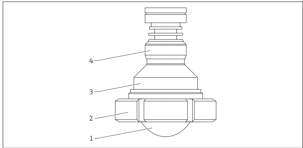
■ 53 Material; Antenne plattiert frontbündig, 80 mm (3 in), Nutmutter DIN11851. Maßeinheit mm (in)
