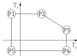
28 Gehäuse 316L; Prozesstemperatur -10 \dots +150 \text{ °C} ( +14 \dots +302 \text{ °F} )
