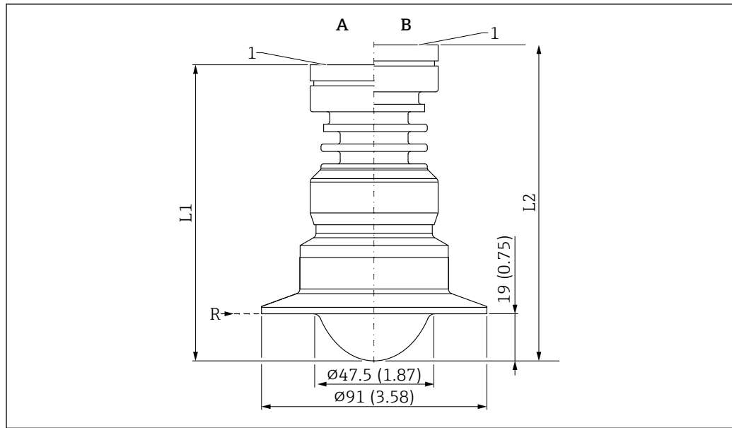
49 Abmessungen Antenne plattiert frontbündig, PTFE, 50 mm (2 in), mit Tri-Clamp DN70-76.1 (3") ISO2852. Maßeinheit mm (in)
