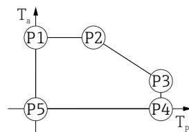
13 Kunststoffgehäuse; Prozesstemperatur 0 \dots +200 \text{ °C} ( +32 \dots +392 \text{ °F} ) bei CSA C/US Zulassung
