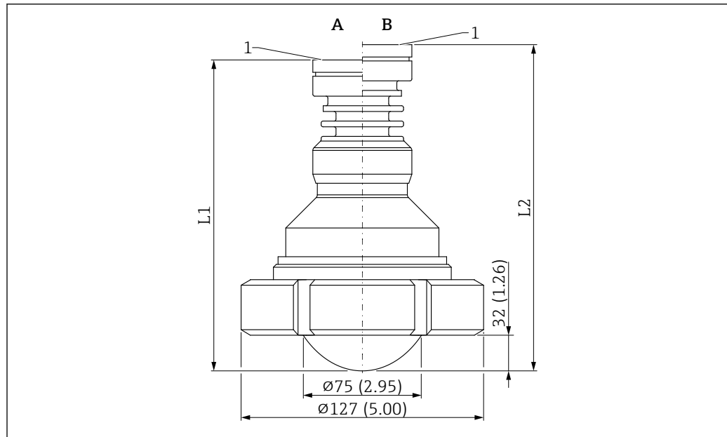
47 Abmessungen Antenne plattiert frontbündig, PTFE, 80 mm (3 in), Nutmutter DIN11851. Maßeinheit mm (in)
