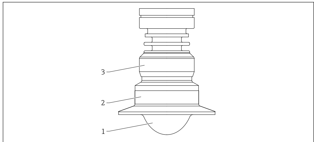
■ 54 Material; Antenne plattiert frontbündig, PTFE, 50 mm (2 in), mit Tri-Clamp ISO2852. Maßeinheit mm (in)
