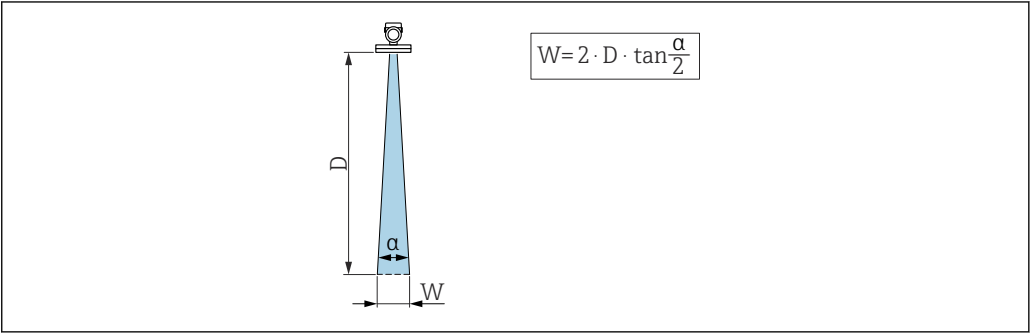
9 Zusammenhang zwischen Abstrahlwinkel \alpha , Distanz D und Kegelseite W
