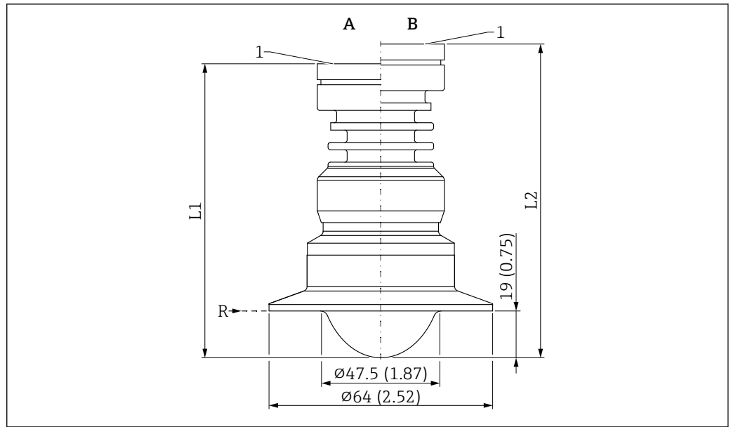
48 Abmessungen Antenne plattiert frontbündig, PTFE, 50 mm (2 in), mit Tri-Clamp DN51 (2") ISO2852. Maßeinheit mm (in)
