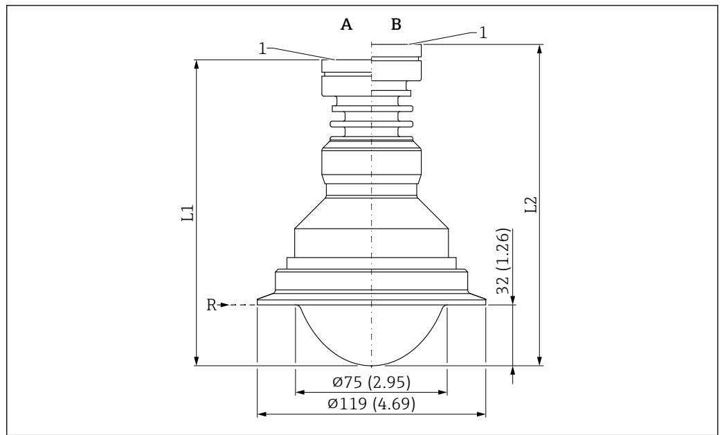
50 Abmessungen Antenne plattiert frontbündig, PTFE, 80 mm (3 in), mit Tri-Clamp DN101.6 (4") ISO2852. Maßeinheit mm (in)
