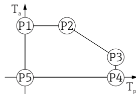
21 Kunststoffgehäuse; Prozesstemperatur 0 \dots +200 \text{ }^{\circ}\text{C} ( +32 \dots +392 \text{ }^{\circ}\text{F} ) bei CSA C/US Zulassung
