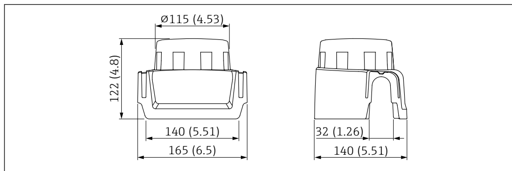
59 Abmessungen. Maßeinheit mm (in)
