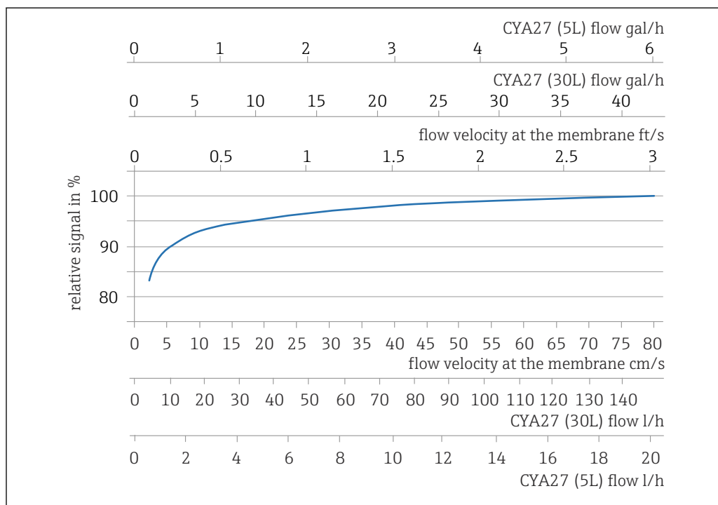
2 Correlação entre slope do eletrodo e velocidade de vazão na vazão volumétrica/membrana no conjunto
