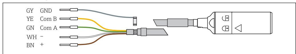
5 Cabo de medição CYK10
