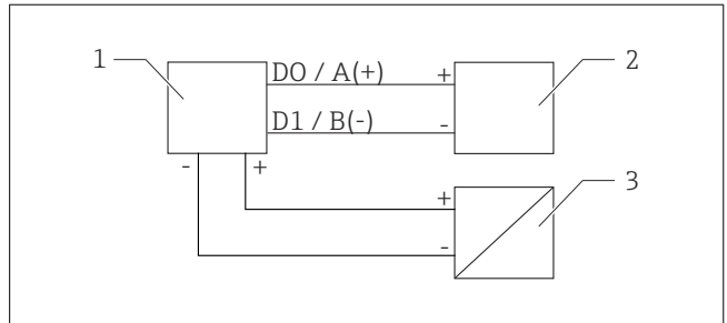
☐ 3 Modbus RS485 연결 계통도
