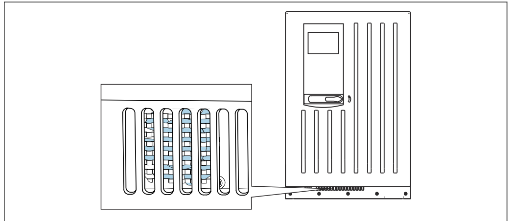
66 Ventola sul modulo di raffreddamento (dietro la griglia di ventilazione)
