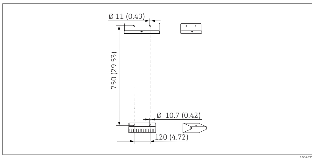
14 Dimensioni dell'unità di supporto Unità ingegneristica mm (in)
