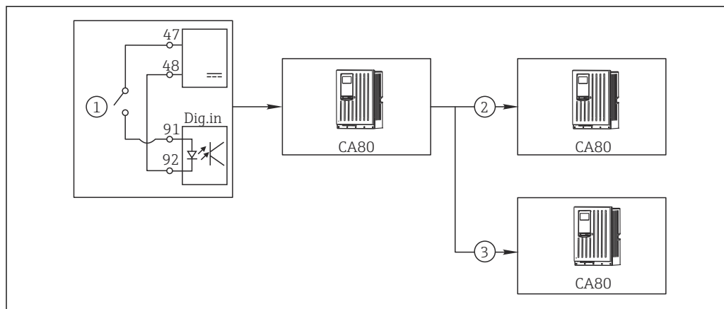
53 Esempio di controllo centralizzato della pulizia
