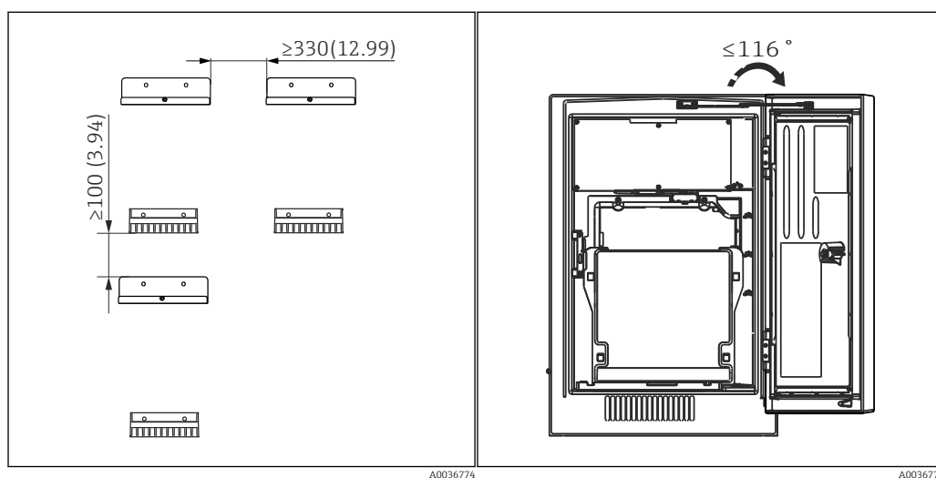
12 Spaziatura minima richiesta per il montaggio. 13 Angolo di apertura massimo Unità ingegneristica mm (in).
