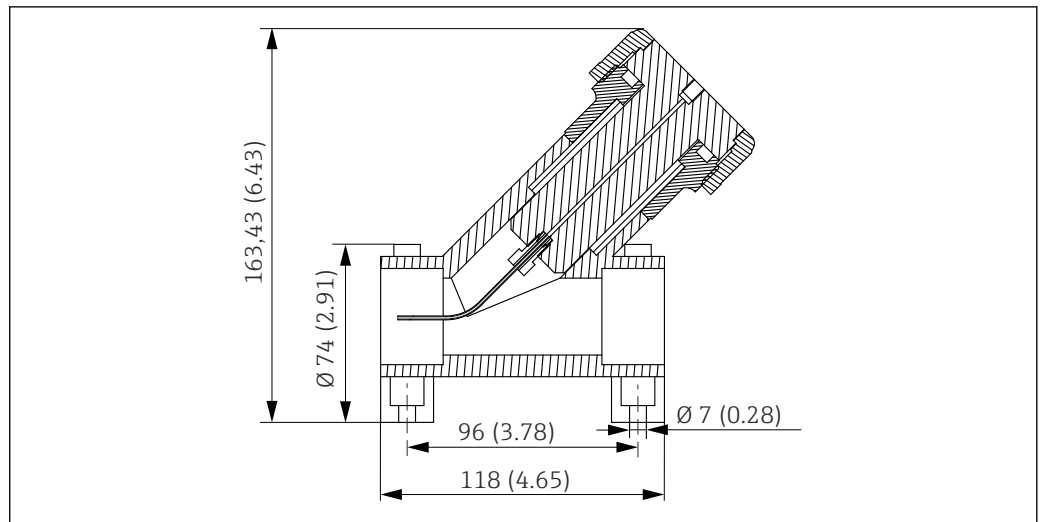
11 Filtro a Y (opzionale), dimensioni in mm (in)
