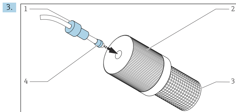
51 Montaggio del filtro di aspirazione (in dotazione) sul tubo flessibile di prelievo
