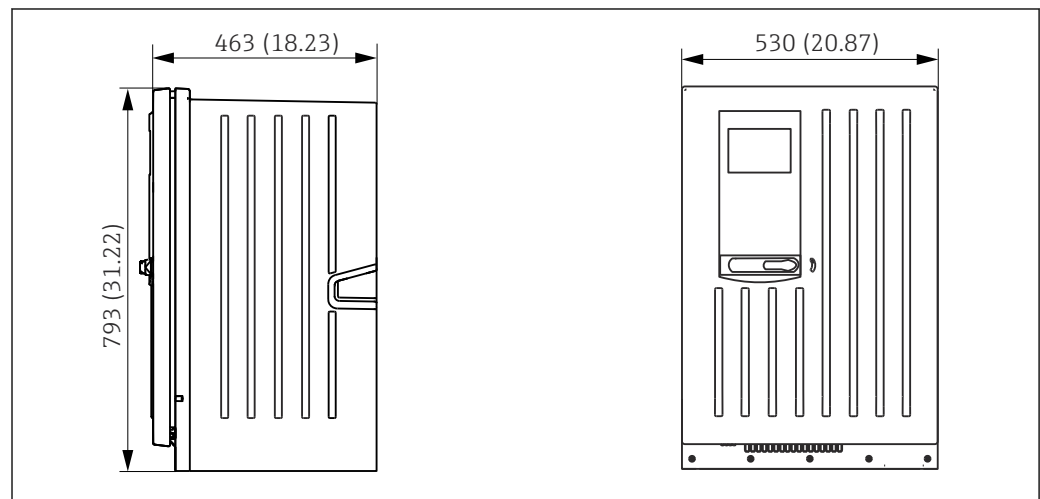
8 Liquiline System CA80 versione chiusa, dimensioni in mm (in)
