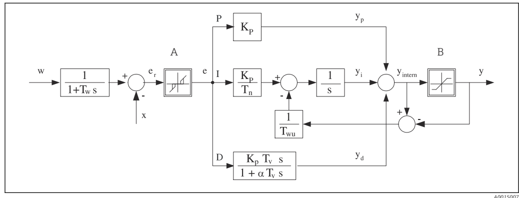
62 Diagramma a blocchi della struttura del controllore
