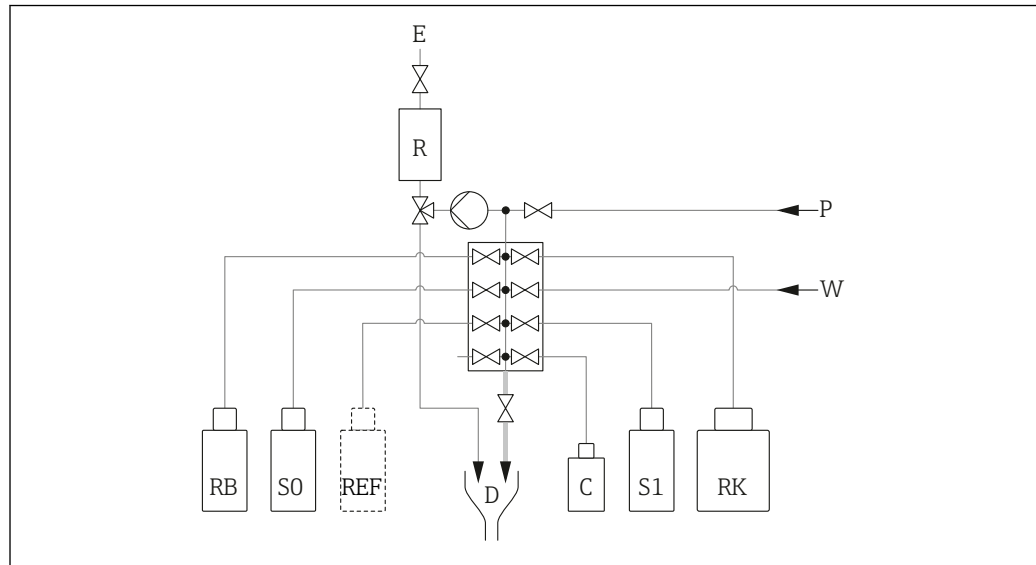
50 Schema di connessione tubi flessibili
