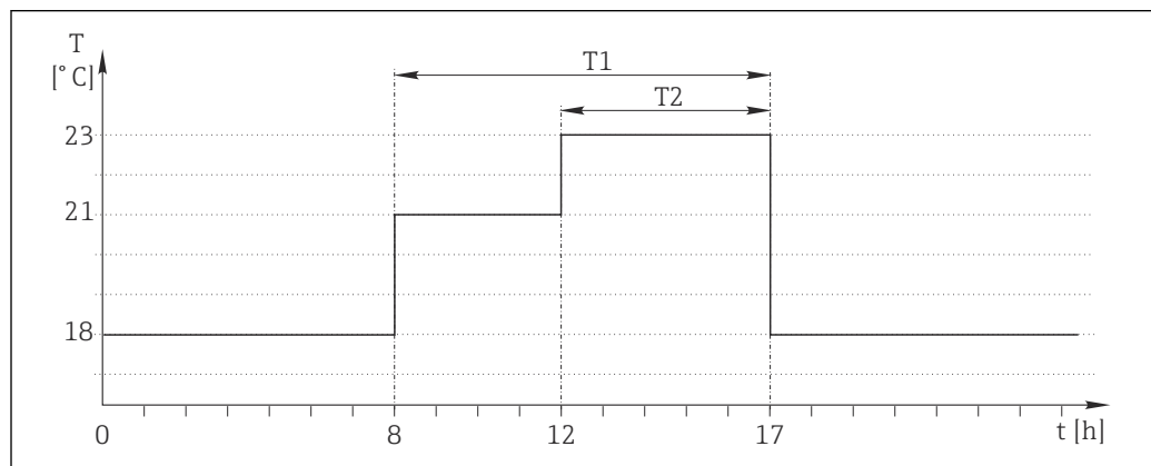
61 Controllo della temperatura basato sul tempo
