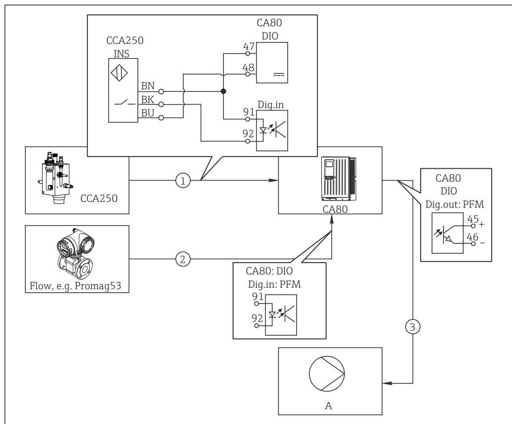
52 Esempio di controllo feedforward del cloro
