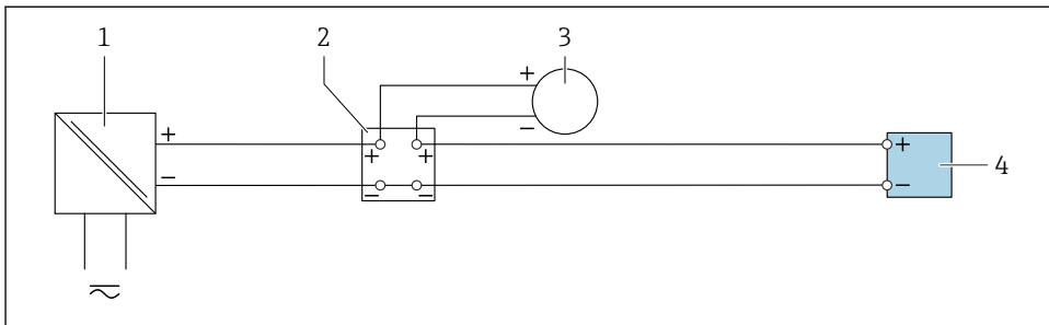
13 Anslutningsexempel för 4 till 20 mA strömingång
