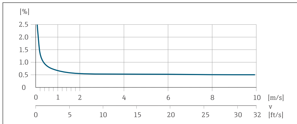
18 Максимальная погрешность измерения в % ИЗМ.
