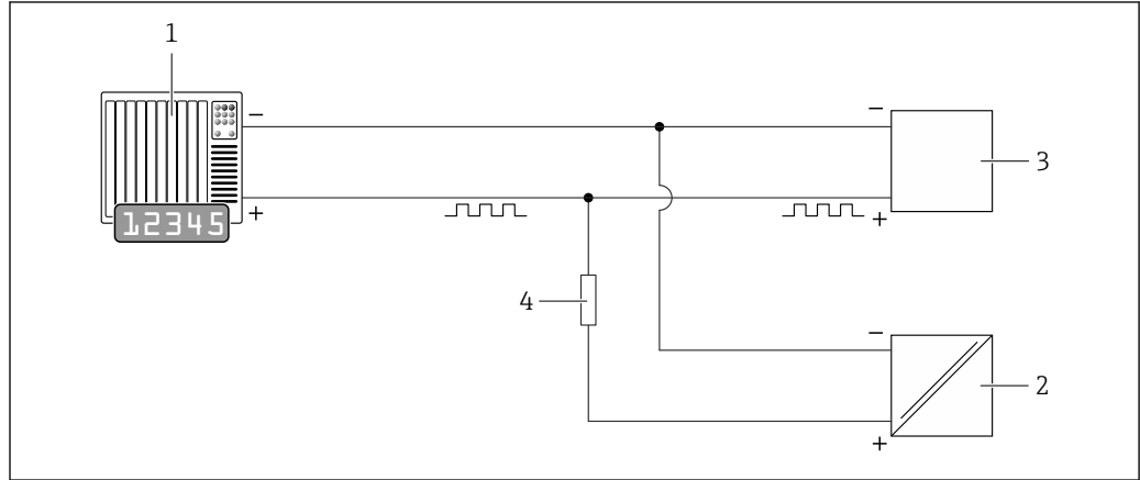
14 Пример подключения для импульсного выхода (пассивного)
