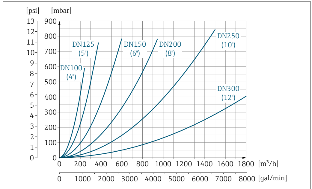
20 Падение давления для DN 100–300 (4–12 дюймов) с кодом заказа «Конструкция», опция С «Фиксированный фланец, суженная измерительная трубка, без входных/выходных участков»
