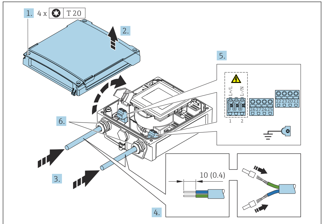
13 Подключение сетевого напряжения и Modbus RS485
