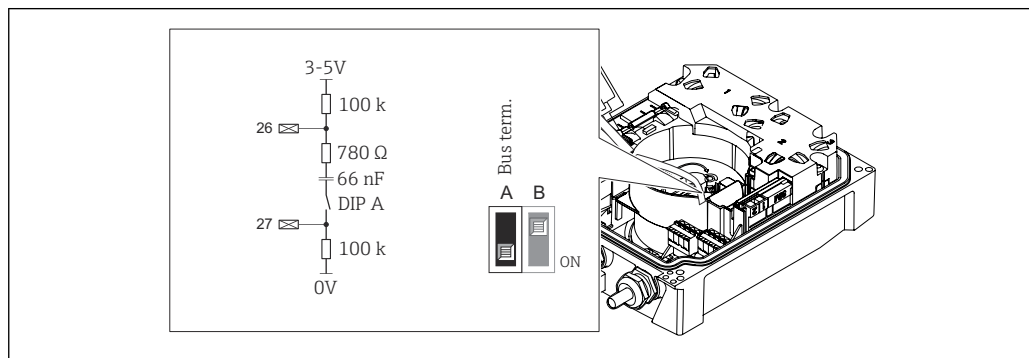
16 Нагрузочный резистор можно активировать с помощью DIP-переключателя на модуле электроники
