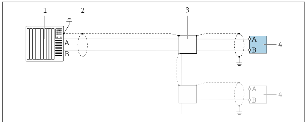
15 Пример подключения для интерфейса Modbus RS485, в невзрывоопасной зоне
