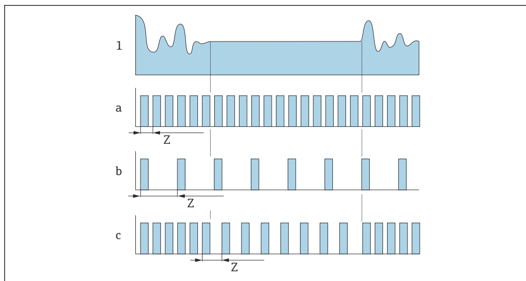
17 Принципы работы различных методов регистрации данных
