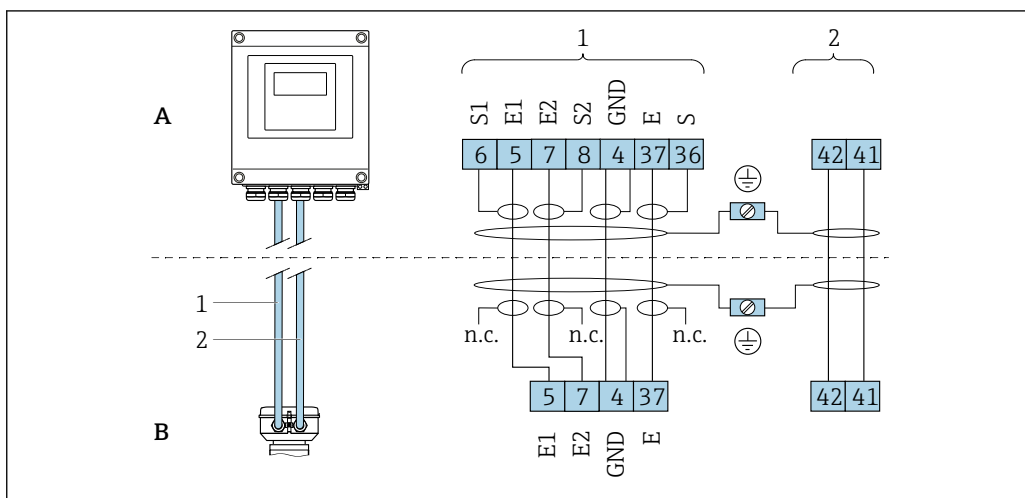
6 Назначение клемм в раздельном исполнении
