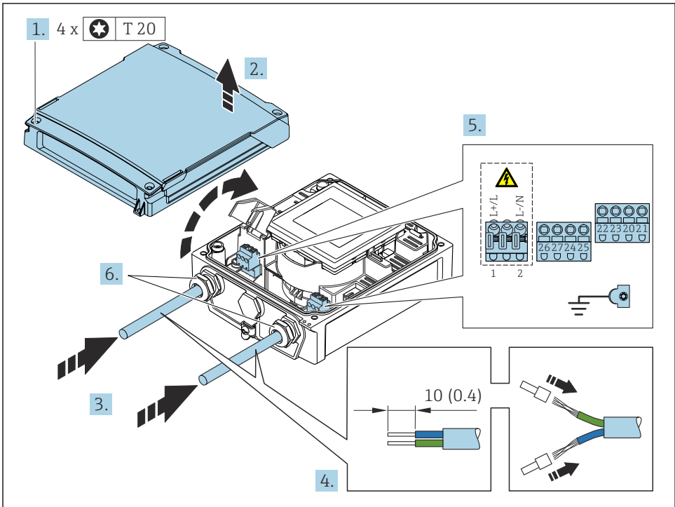
图 7 连接电源和 Modbus RS485
