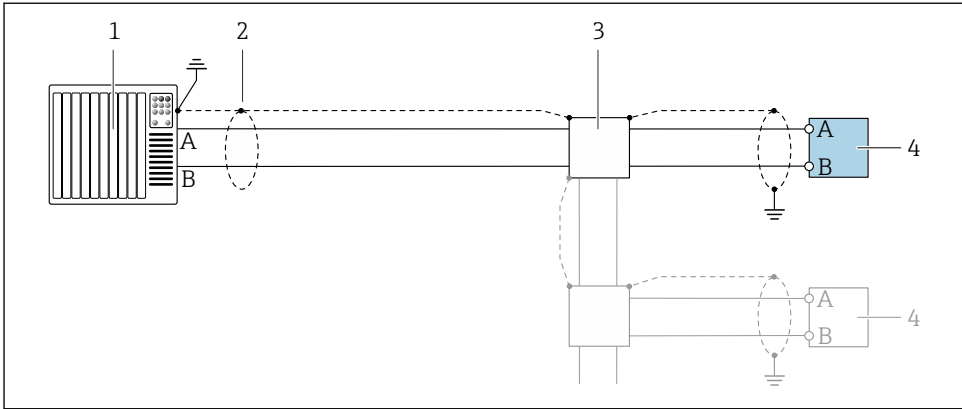
图 12 接线示例: Modbus RS485, 非危险区
