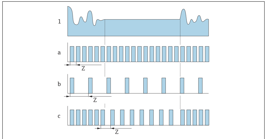
图 5 不同数据记录方式的工作原理
