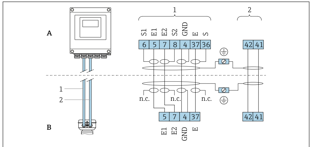
图 6 分体型仪表的接线端子分配
