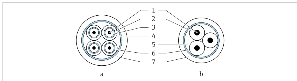
图 9 电缆截面图
