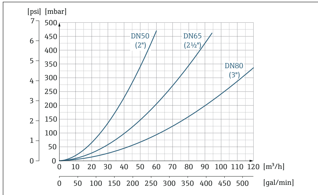
图 24 压损：适用口径 DN 50...80 (2...3")；订购选项“设计”，选型代号 C “固定法兰，缩径测量管，无前后直管段长度要求”
