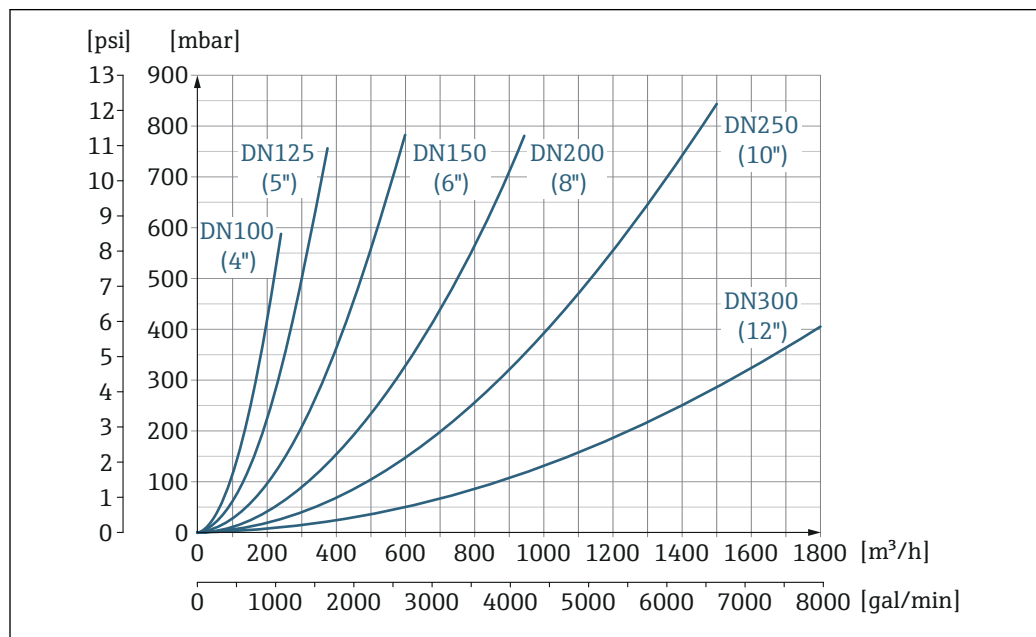
图 25 压损：适用口径 DN 100...300 (4...12")；订购选项“设计”，选型代号 C “固定法兰，缩径测量管，无前后直管段长度要求”
