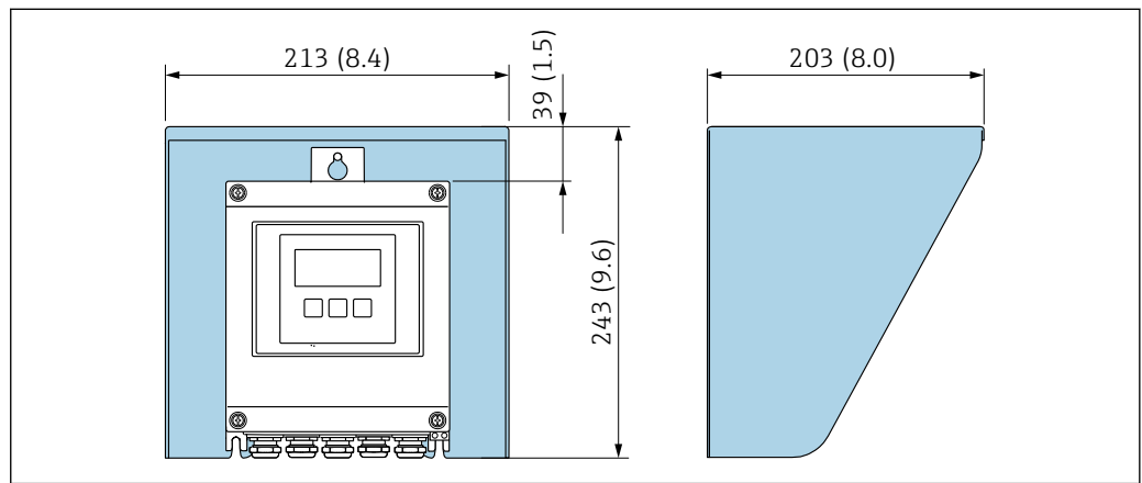
图 26 防护罩的外形尺寸示意图; 单位: mm (in)
