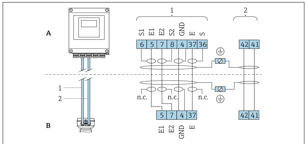
4 Assegnazione dei morsetti per la versione separata
