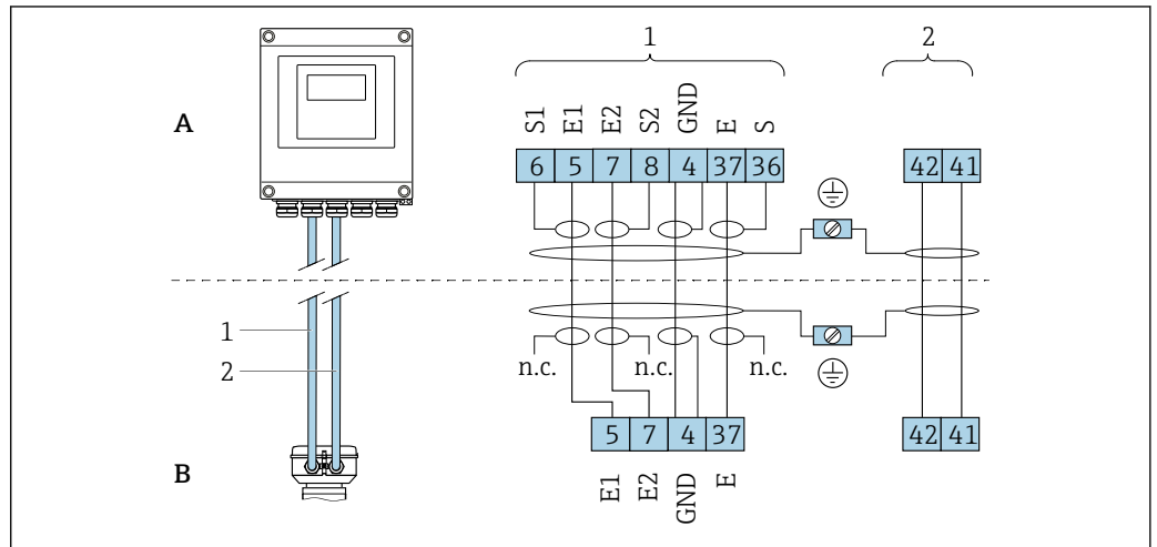
6 Assegnazione dei morsetti per la versione separata
