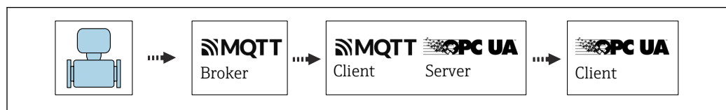
2 Connessione radio cellulare tramite broker MQTT, server OPC-UA e crittografia TLS.
