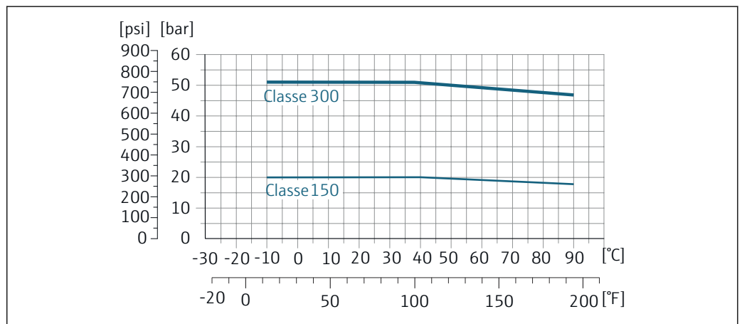
18 Materiale della connessione al processo: acciaio al carbonio
