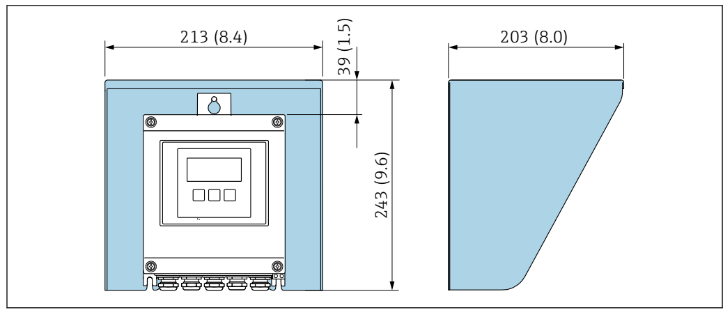
14 Tettuccio di protezione dalle intemperie, unità ingegneristiche mm (in)
