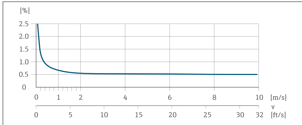
10 Errore di misura massimo in % v.i.
