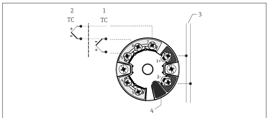
11 Trasmittitore per montaggio da testa TMT8x (doppio ingresso sensore)
