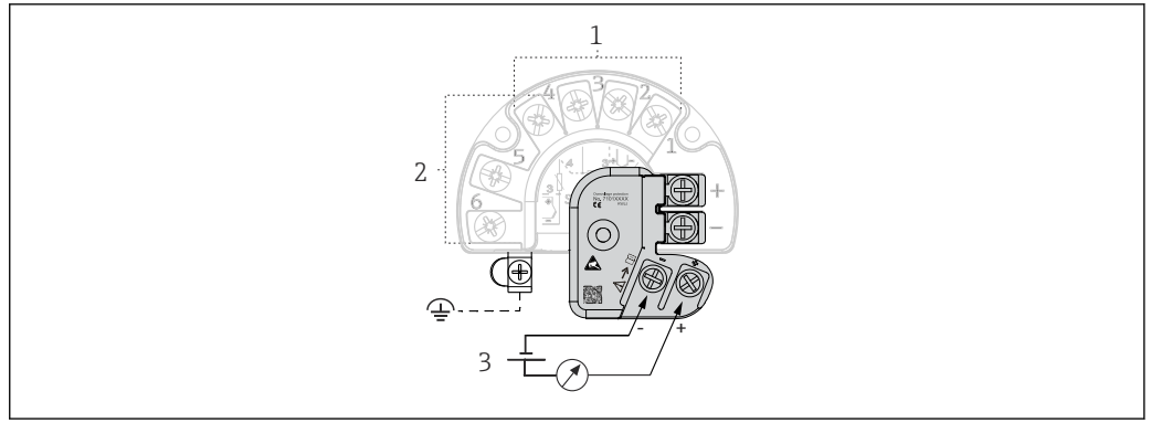
14 Collegamento elettrico della protezione da sovratensione
