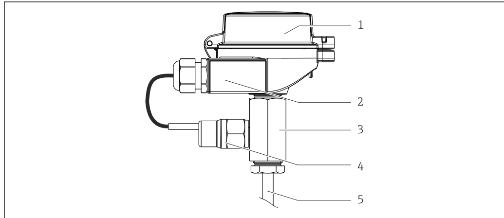
27 Collo di estensione con seconda tenuta di processo
