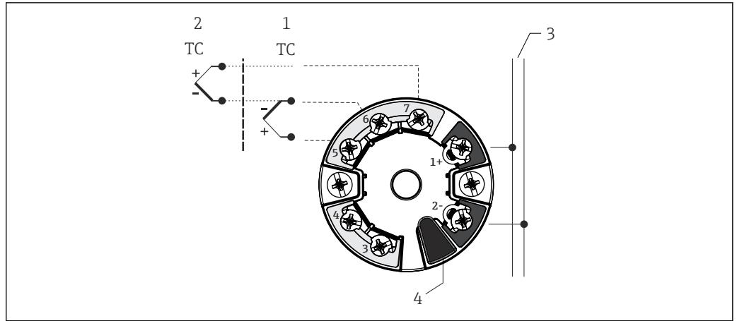
图 7 TMT8x 模块化温度变送器 (双路传感器输入)
