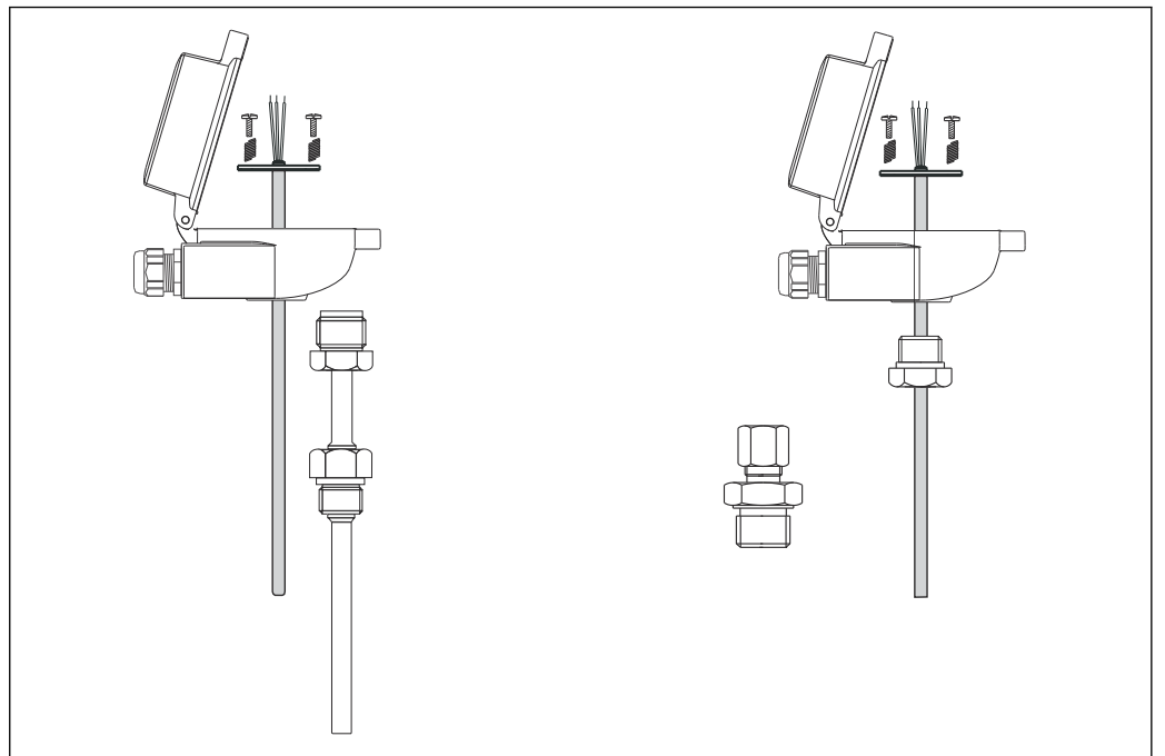
图 9 常规安装选项: 在带有保护套管的安装支架中 (左), 直接测量 (右)
