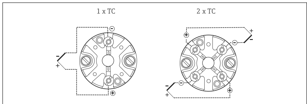
图 5 已安装陶瓷端子接线块
