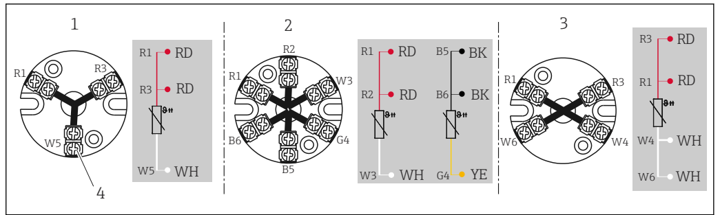
图 1 安装的陶瓷端子接线块
