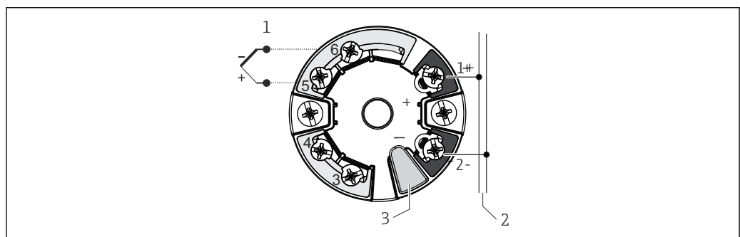
图 6 TMT7x 模块化温度变送器 (单输入通道)
