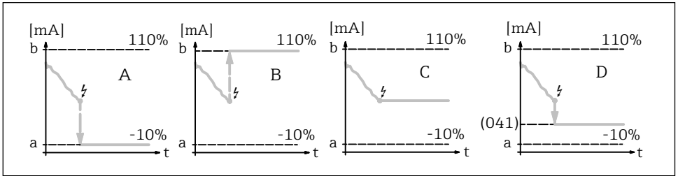
14 Gedrag van de huidige uitgang bij een fout
