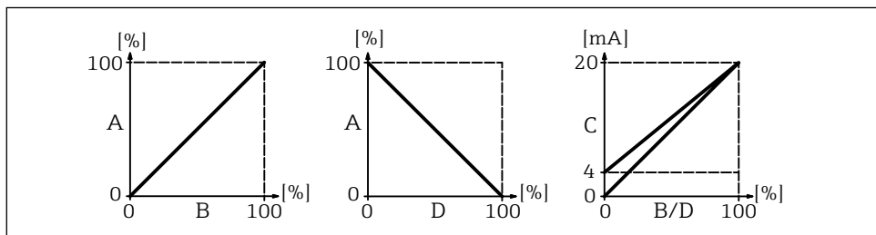
13 Gedrag van de huidige uitgang
