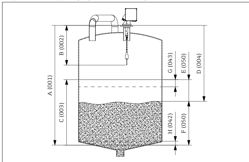
11 Parameters van de basisopstelling
