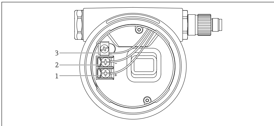
17 Zaciski połączeniowe i zacisk uziemienia w przedziale podłączeniowym
