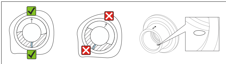
9 Adapter do spawania z otworem spustowym
