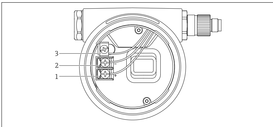
17 Соединительные клеммы и клемма заземления в клеммном отсеке
