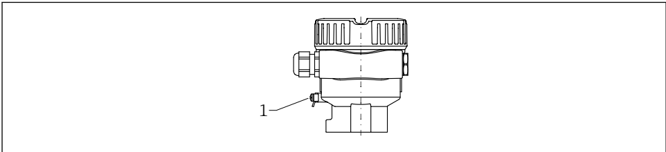
1 Клемма заземления для подключения линии выравнивания потенциалов
