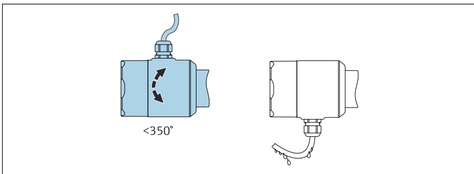
13 Корпус без стопорного винта с ниспадающей каплеуловительной кабельной петлей
