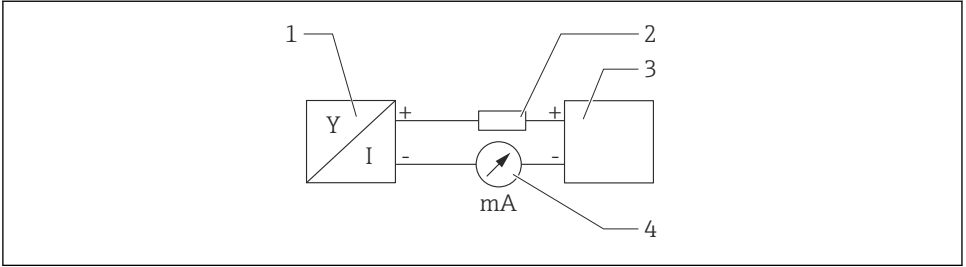
16 HART 연결 계통도
