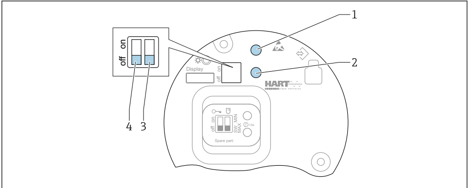
☞ 20 FEL60H 기판의 작동 키 및 DIP 스위치
