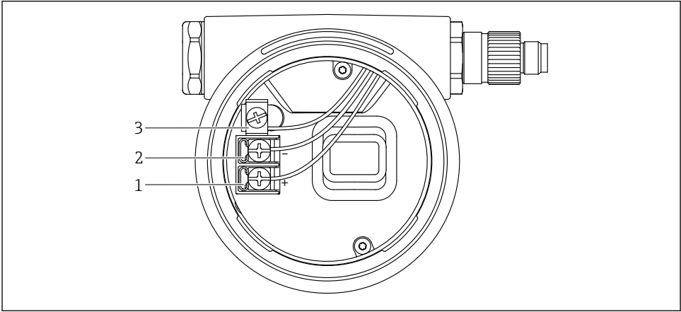
☐ 17 연결부의 연결 단자 및 접지 단자
