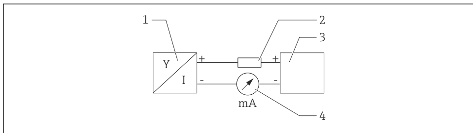
15 Schemat blokowy podłączenia wersji HART
