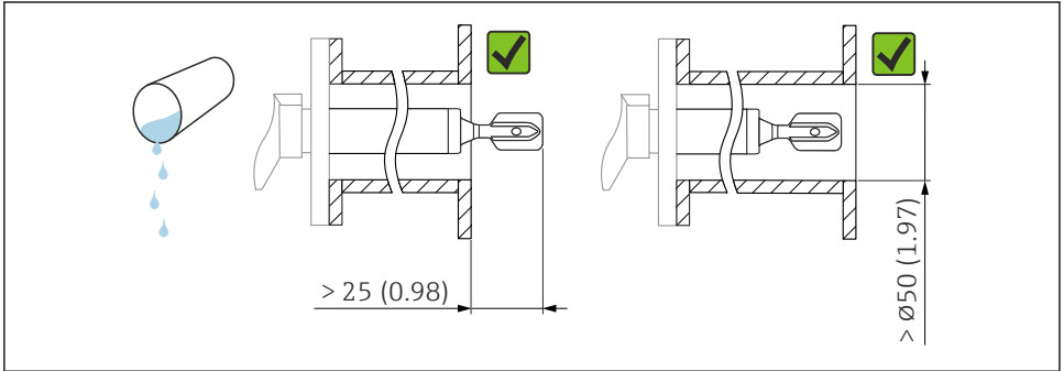
5 Przykład montażu w cieczech o małej lepkości. Jednostka miary mm (in)
