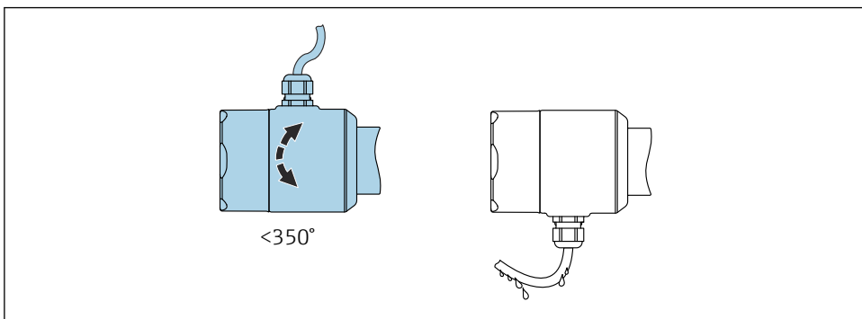
12 Корпус без стопорного винта с ниспадающей каплеуловительной кабельной петлей
