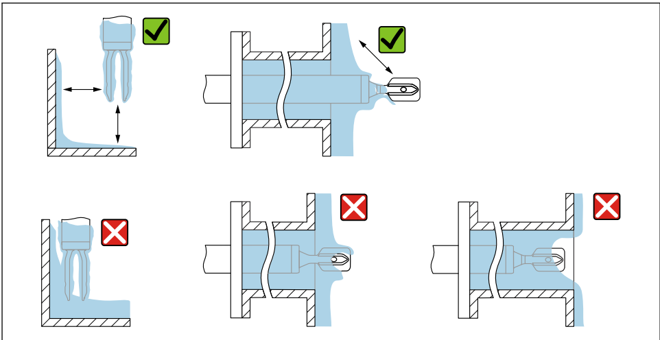
☞ 6 고점성 프로세스 유체용 설치 예
