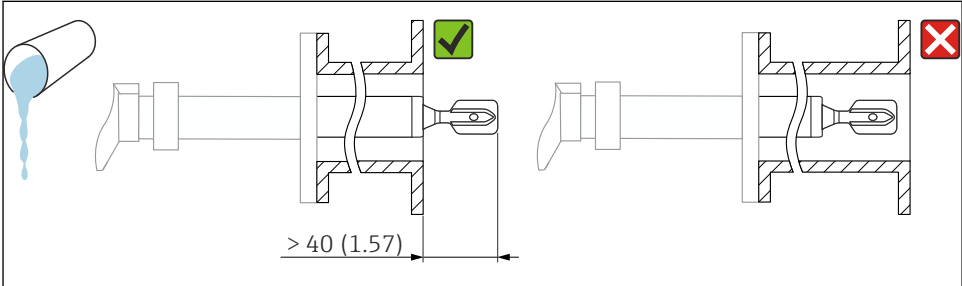
☞ 5 고점성 액체용 설치 예. 측정 단위 mm (in)
