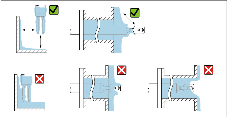
6 Exemple de instalare pentru un mediu de proces deosebit de vâscos
