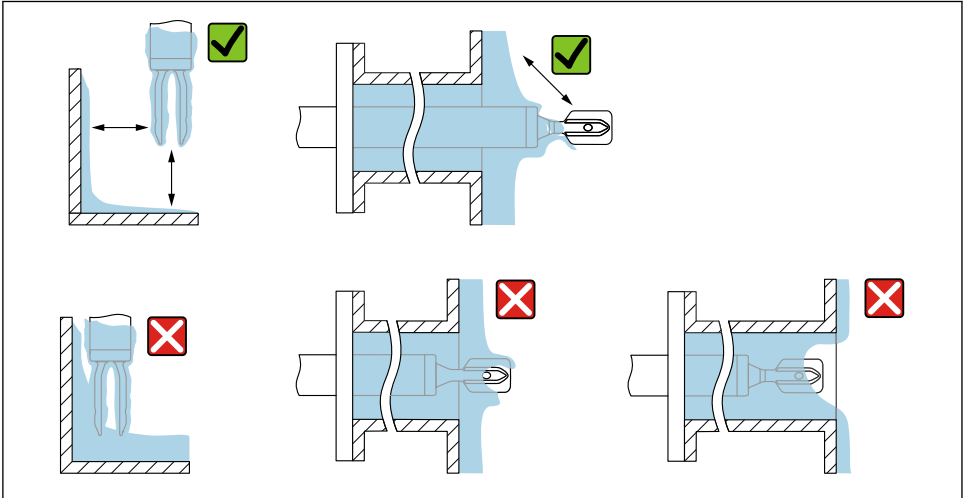
6 Exemplos de instalação para um meio de processo altamente viscoso
