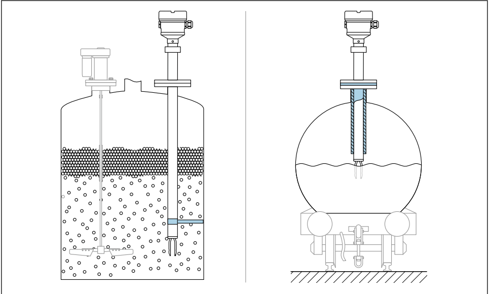
8 Exemplos de suporte em casos de carga dinâmica
