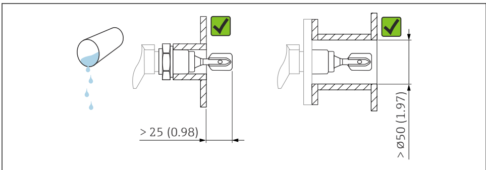
3 安装实例: 测量低粘度液体。测量单位 mm (in)
