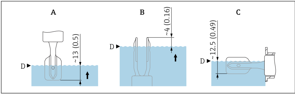
2 常见开关点。测量单位 mm (in)
