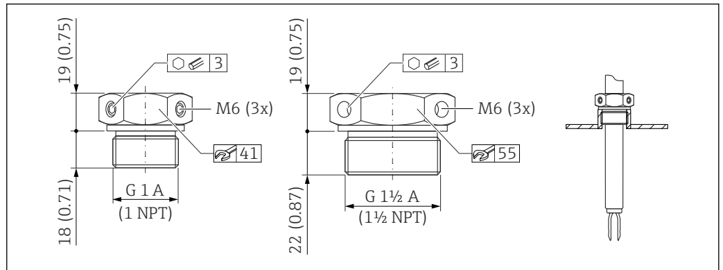
图 32 常压滑动套管 p_e = 0 bar (0 psi)。测量单位 mm (in)
