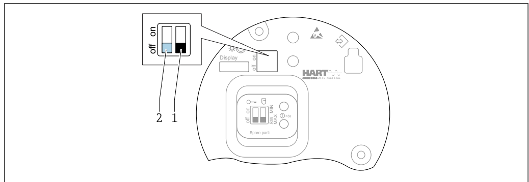
图 27 FEL60H 电子插件上的 DIP 开关的功能
