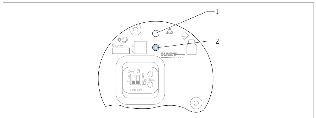
图 22 FEL60H 电子插件上的操作按键
