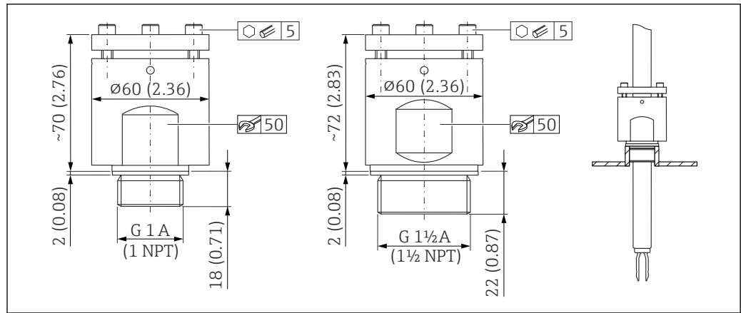
图 33 高压滑动套管。测量单位 mm (in)
