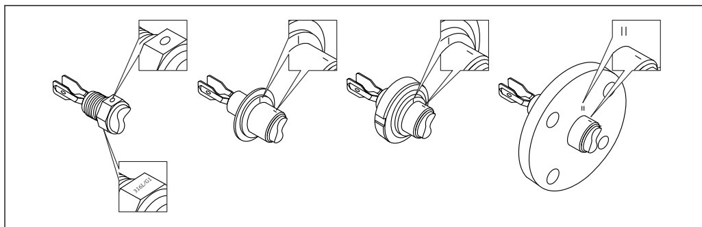
11 Posizione della forcella vibrante quando installato orizzontalmente nel silo utilizzando il contrassegno
