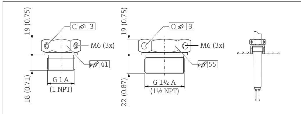
32 Manicotti scorrevoli per il funzionamento non pressurizzato p_e = 0 bar (0 psi). Unità di misura mm (in)
