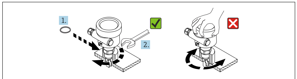
13 Прикручивание прибора
