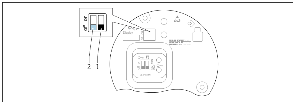
☑ 27 Функции DIP-переключателей на электронной вставке FEL60H
