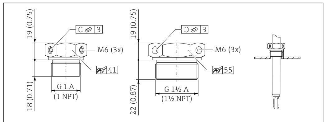
32 Скользящие муфты для использования при отсутствии избыточного давления, p_e = 0 бар (0 фунт/кв. дюйм). Единица измерения мм (дюйм)
