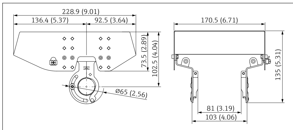
29 Защитный козырек от погодных явлений для корпуса с двумя отсеками. Единица измерения мм (дюйм)
