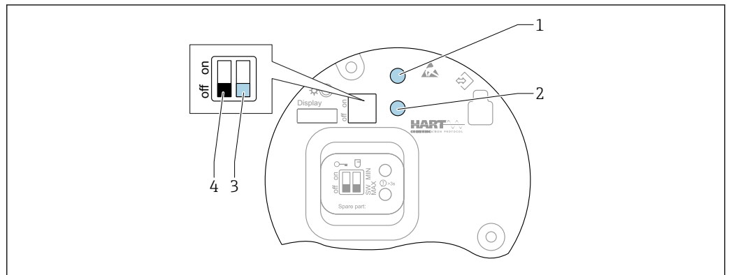
Fig. 27 Teclas de operação e minisseletores na unidade eletrônica FEL60H
