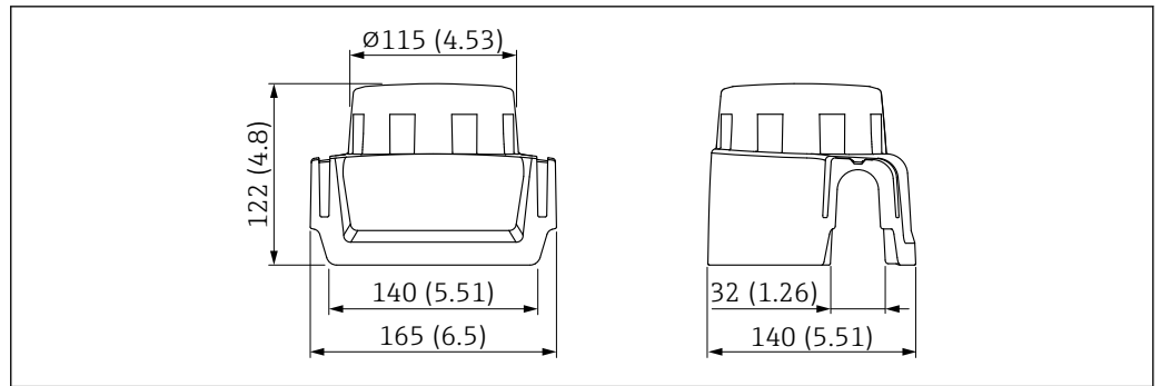
31 Capa protetora para invólucro de alumínio com compartimento único. Unidade de medida mm (in)
