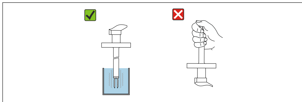
25 Teste funcional do diapásão
