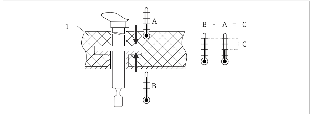
4 Diferença de temperatura entre o lado exterior e interior da flange
