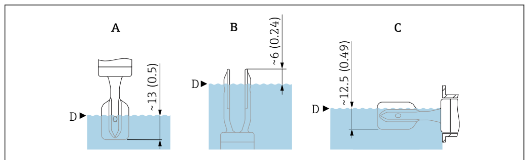
5 Pontos de comutação típicos, diapasão revestido em plástico (ECTFE, PFA). Unidade de medida mm (in)
