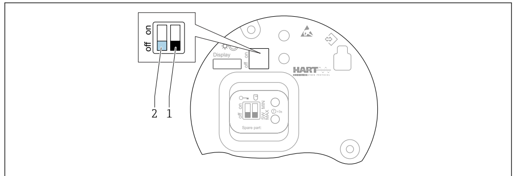
28 Funções das minisseletoras na unidade eletrônica FEL60H
