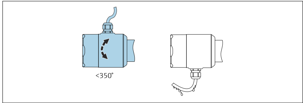
14 Invólucro sem parafuso de travamento com loop de gotejamento
