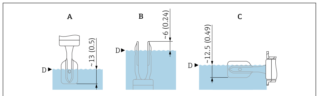
5 Points de détection typiques, fourche vibrante revêtue de plastique (ECTFE, PFA). Unité de mesure mm (in)
