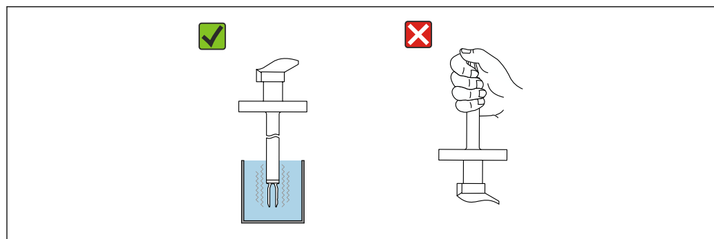
25 Test de fonctionnement de la fourche vibrante
